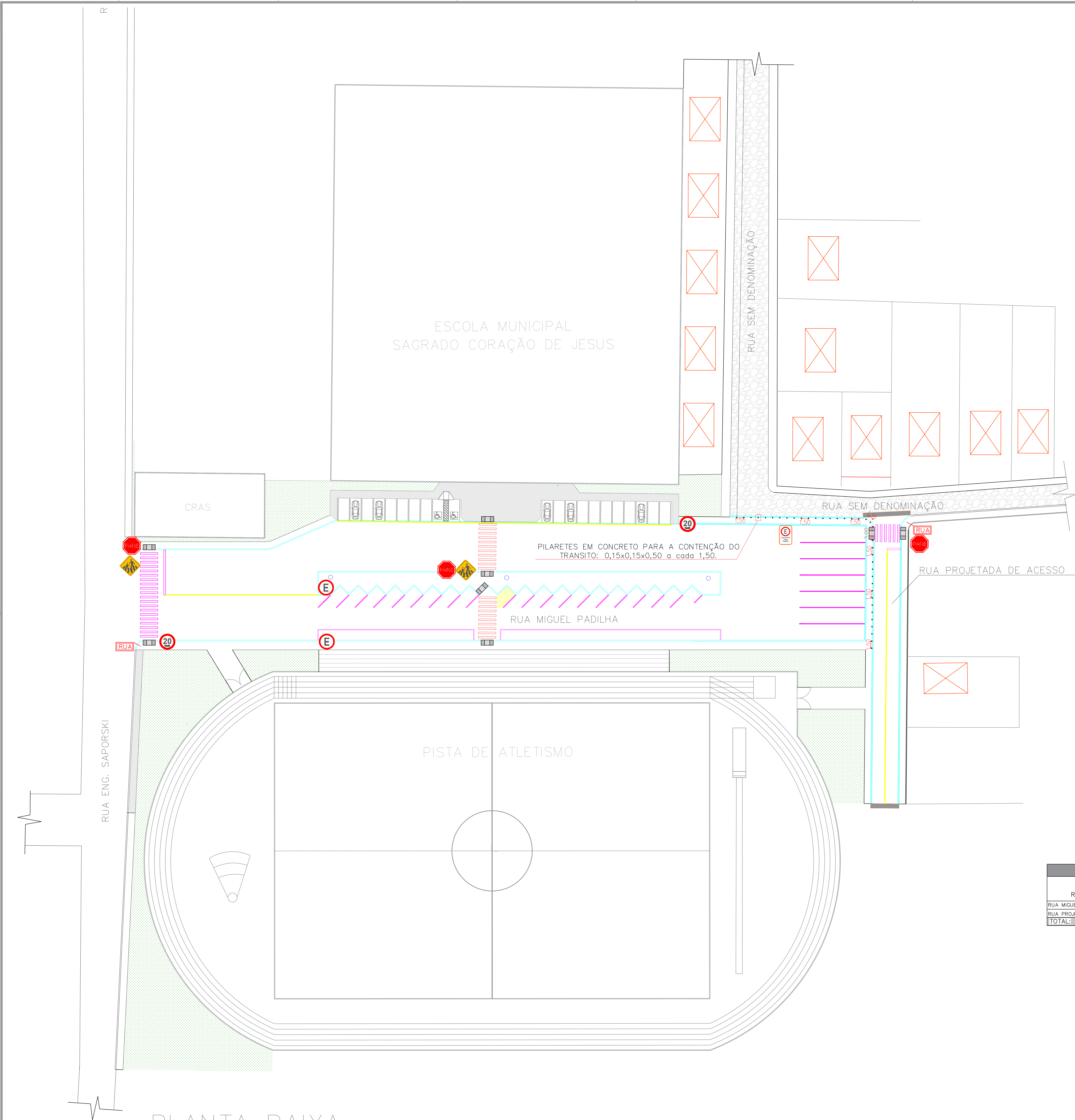
PLANTA BAIXA SINALIZAÇÃO SEM ESCALA
