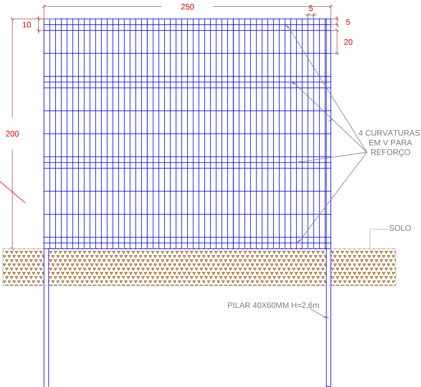
DETALHE CERCA ESC. 1/20
