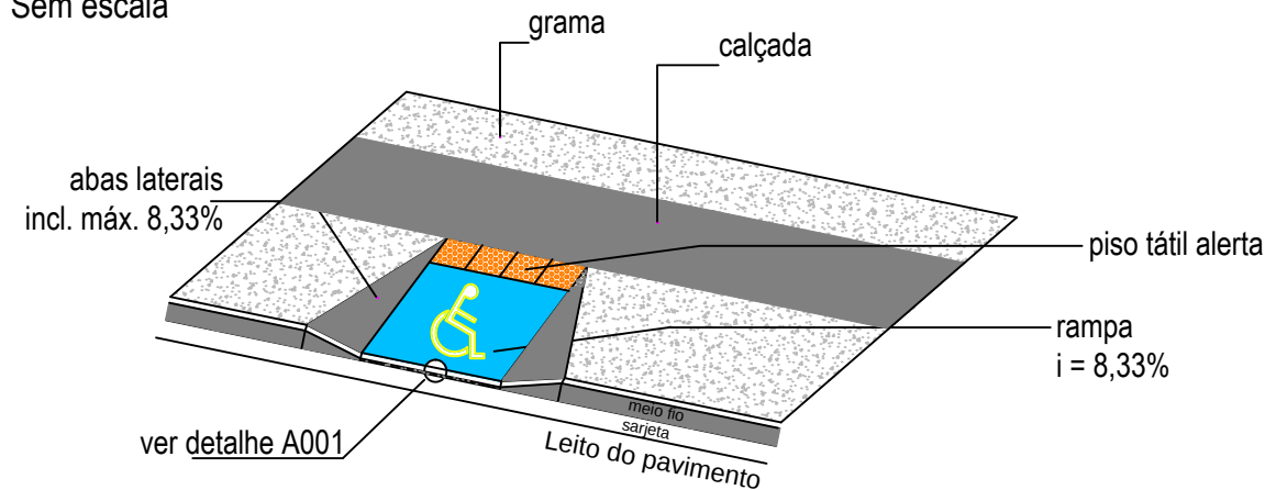
Detalhe "B" Perspectiva
