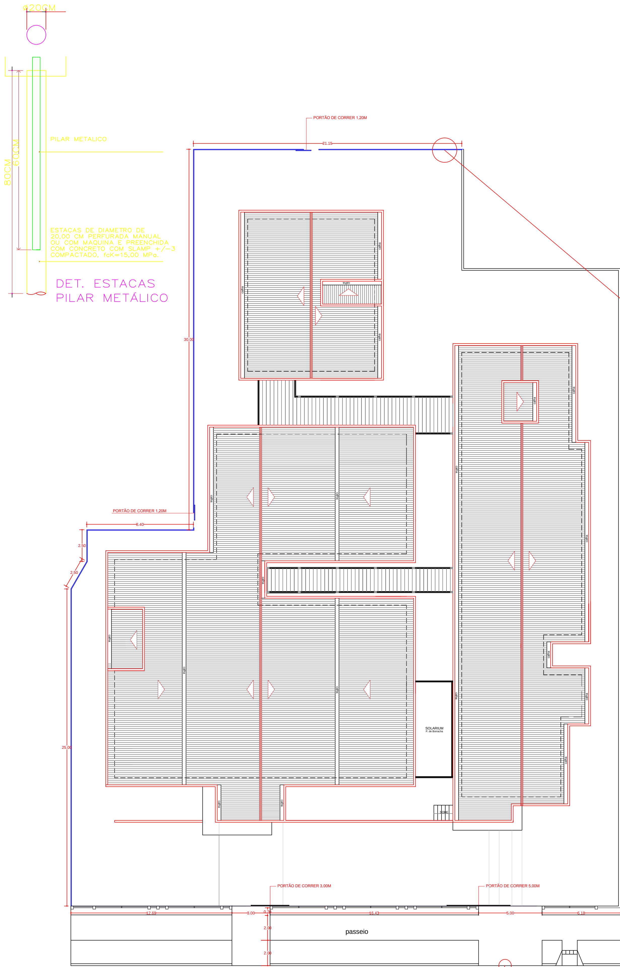
PLANTA DE IMPLANTAÇÃO Esc.: 1:150
