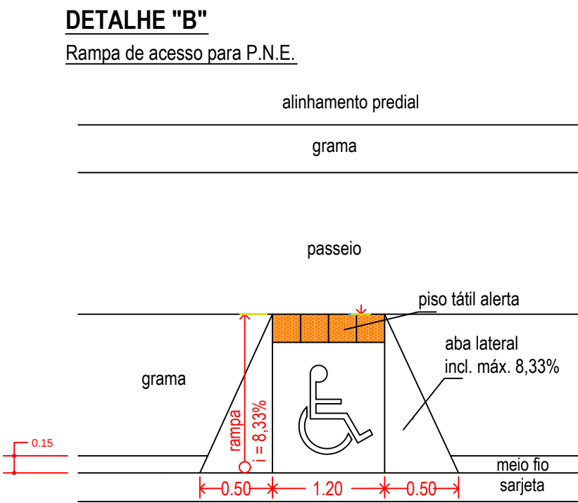
Planta Baixa Sem escala
