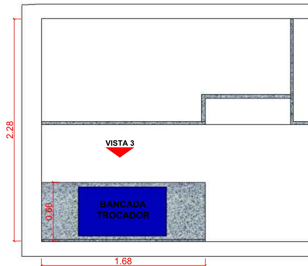
PLANTA BAIXA BANHEIRO TROCADOR
