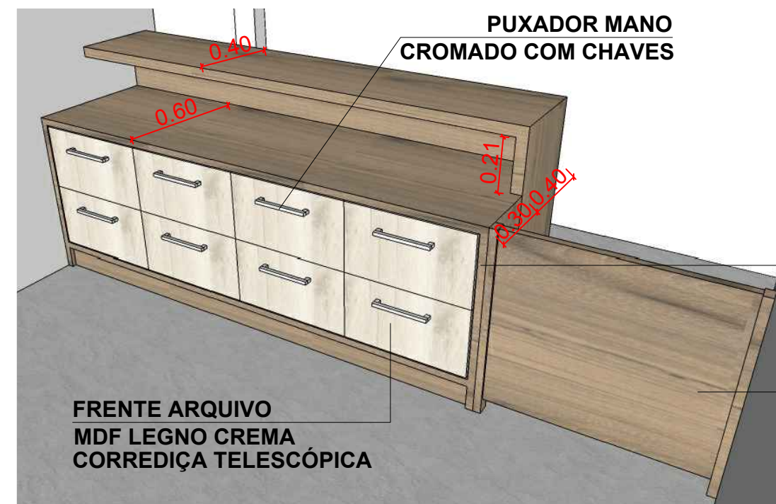
2. PERSPECTIVA BALCÃO DE ATENDIMENTO
