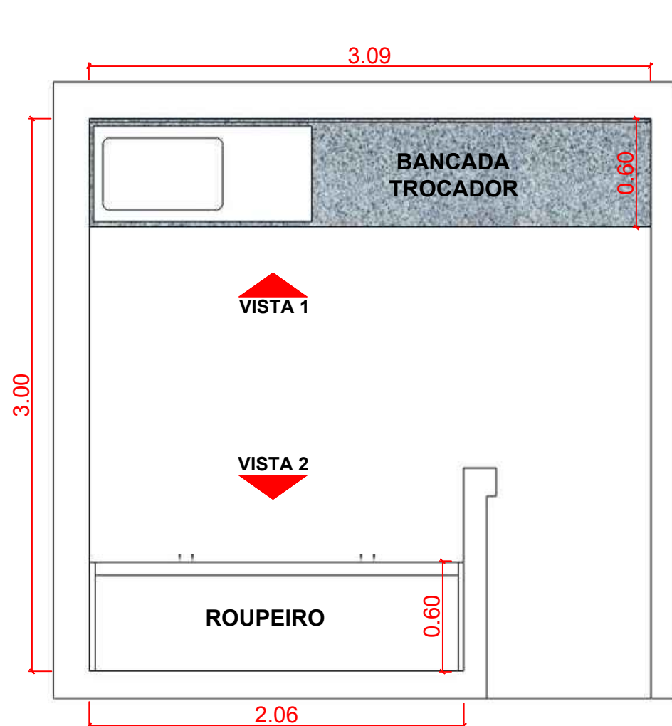
PLANTA BAIXA
