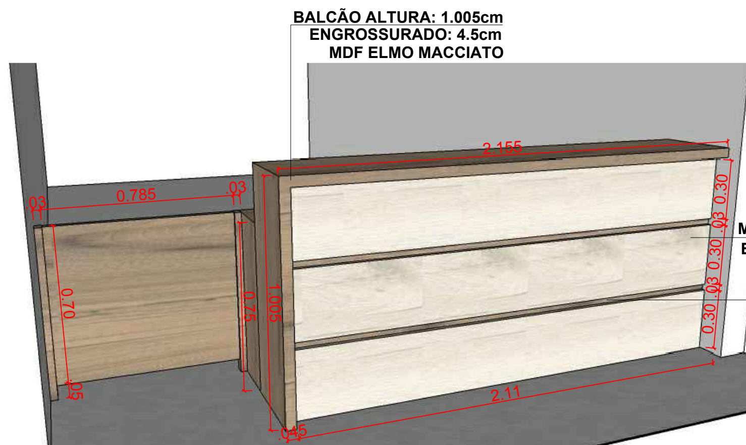
3. VISTA FRONTAL - BALCÃO DE ATENDIMENTO
