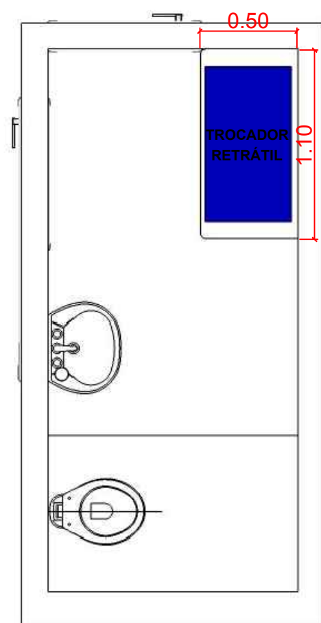
PLANTA BAIXA BANHEIRO TROCADOR RETRÁTIL
