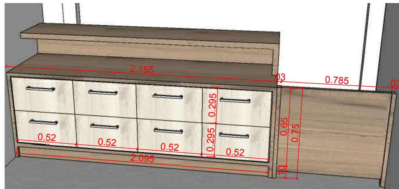
1. PERSPECTIVA BALCÃO DE ATENDIMENTO
