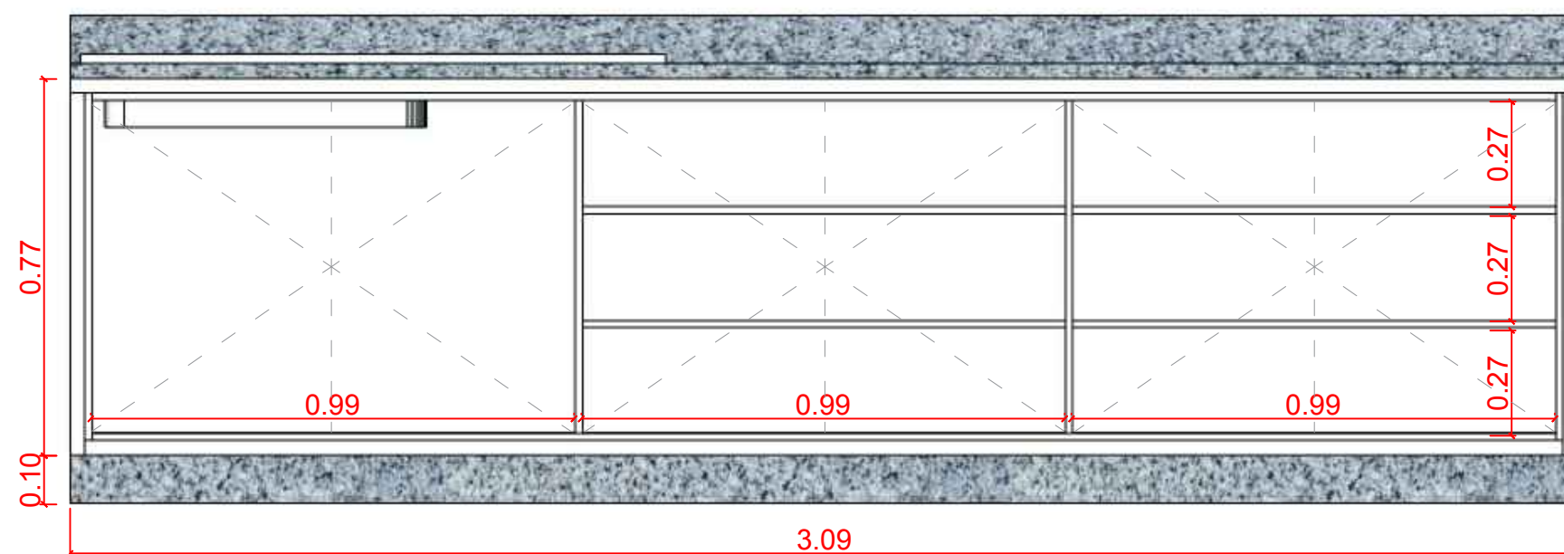
VISTA FRONTAL - TROCADOR INTERNO
