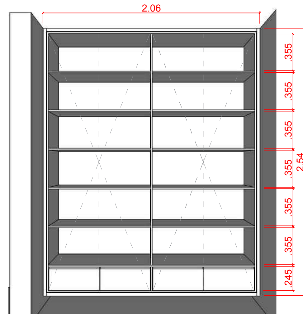
PERSPECTIVA - ROUPEIRO INTERNO
