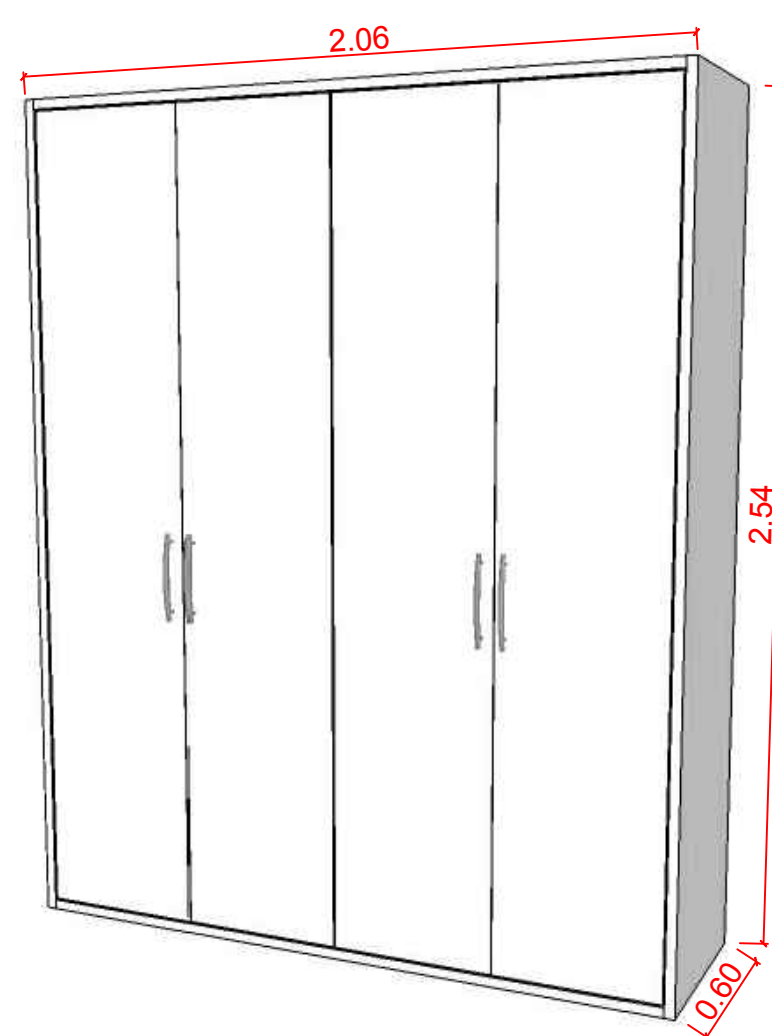
PERSPECTIVA - ROUPEIRO
