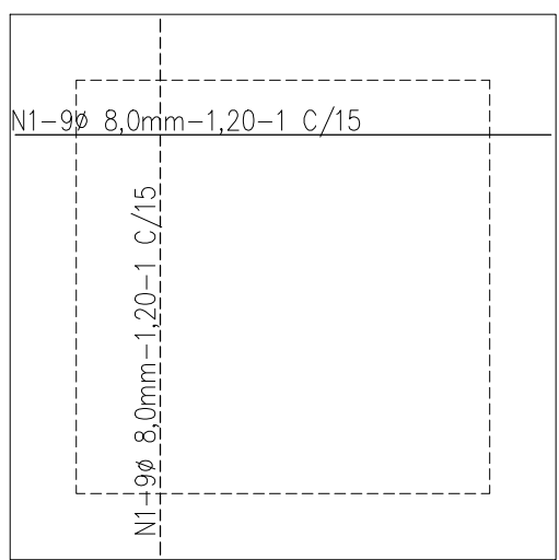
TAMPA ESCALA 1/25
