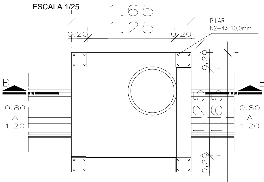
LAJE INFERIOR ESCALA 1/25
