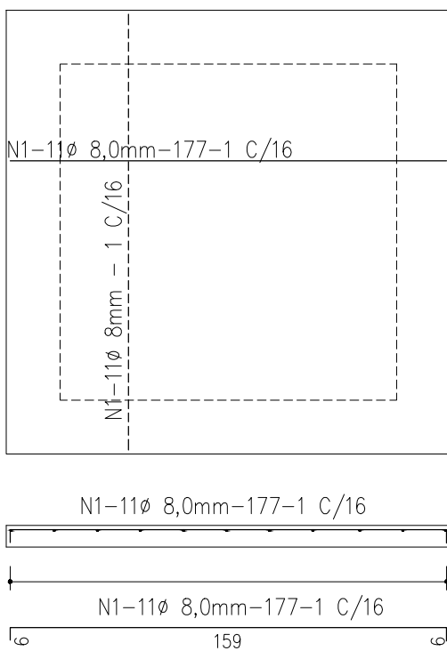
LAJE INFERIOR ESCALA 1/25
