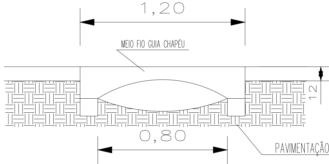
DETALHE DO MEIO-FIO ESCALA 1/12,5
