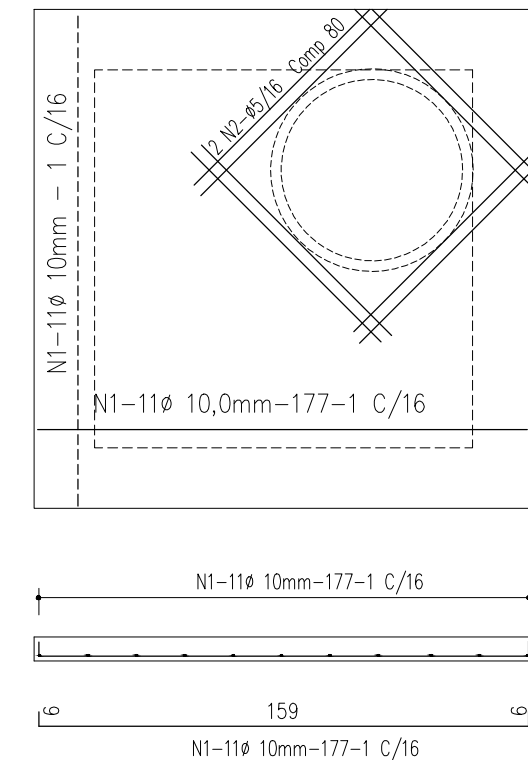
LAJE SUPERIOR ESCALA 1/25
