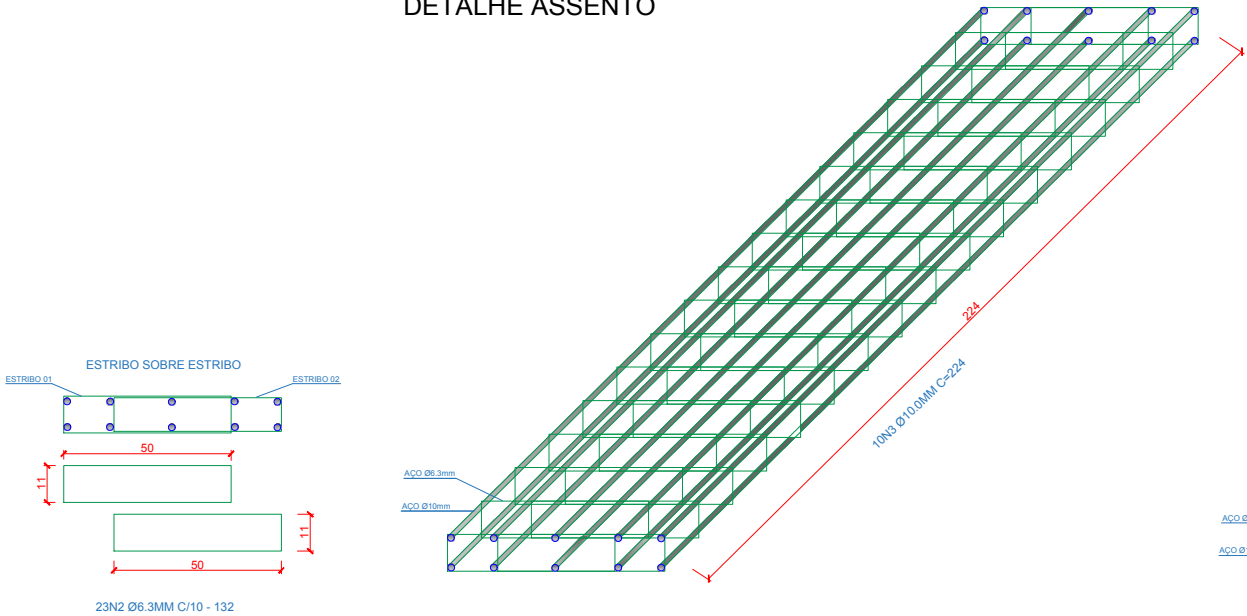
DETALHE ASSENTO
