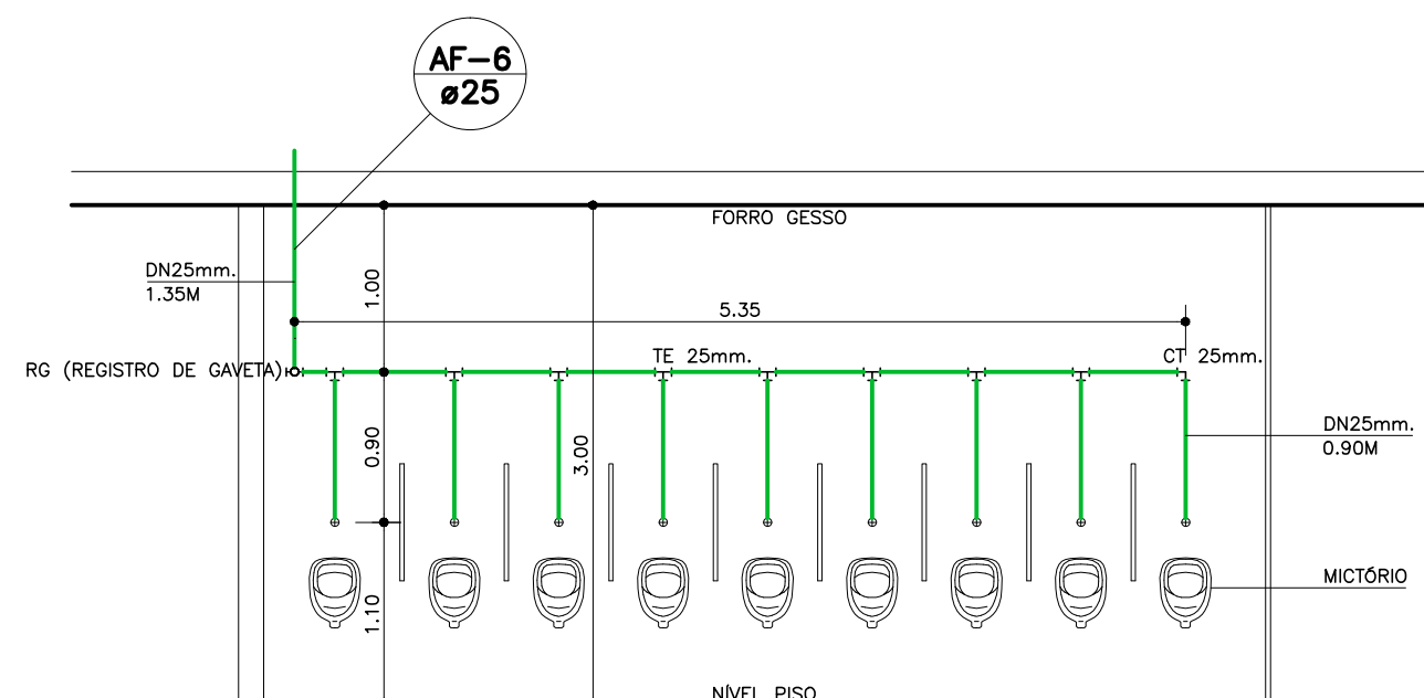
CORTE A - HIDRAULICO (REDE DE AGUA) ESCALA: 1:50
