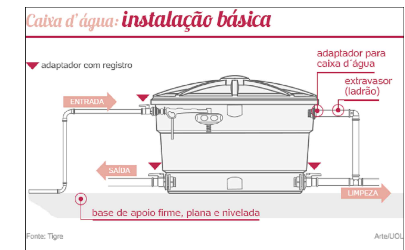
IMAGEM ILUSTRATIVA - DETALHE INSTALAÇÃO
