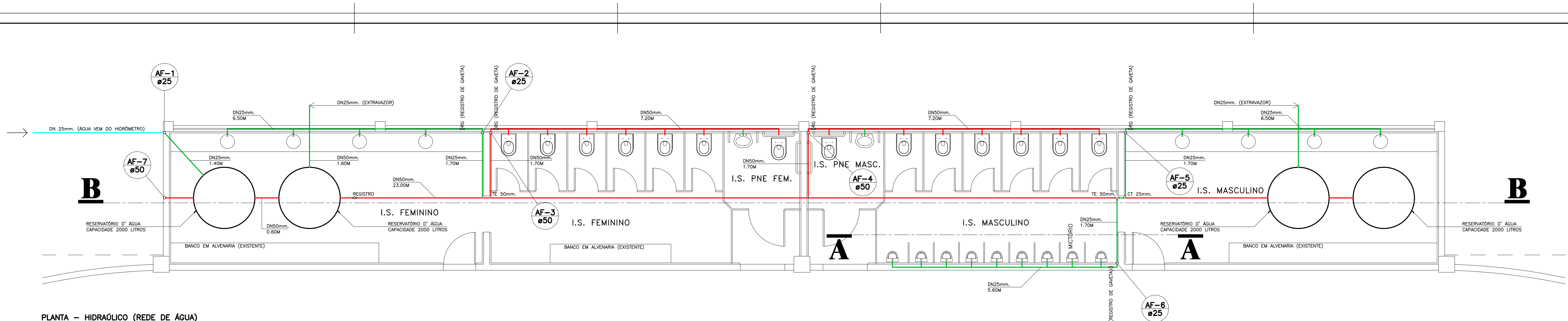
PLANTA - HIDRAULICO (REDE DE AGUA) ESCALA: 1:50
