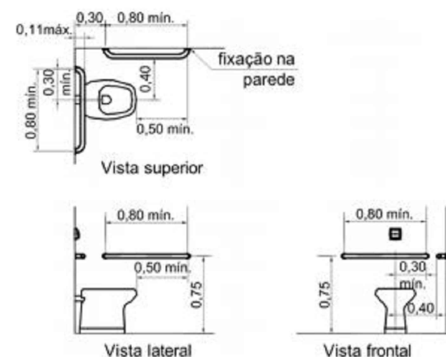
DETALHE - BACIA SANITÁRIA PNE
