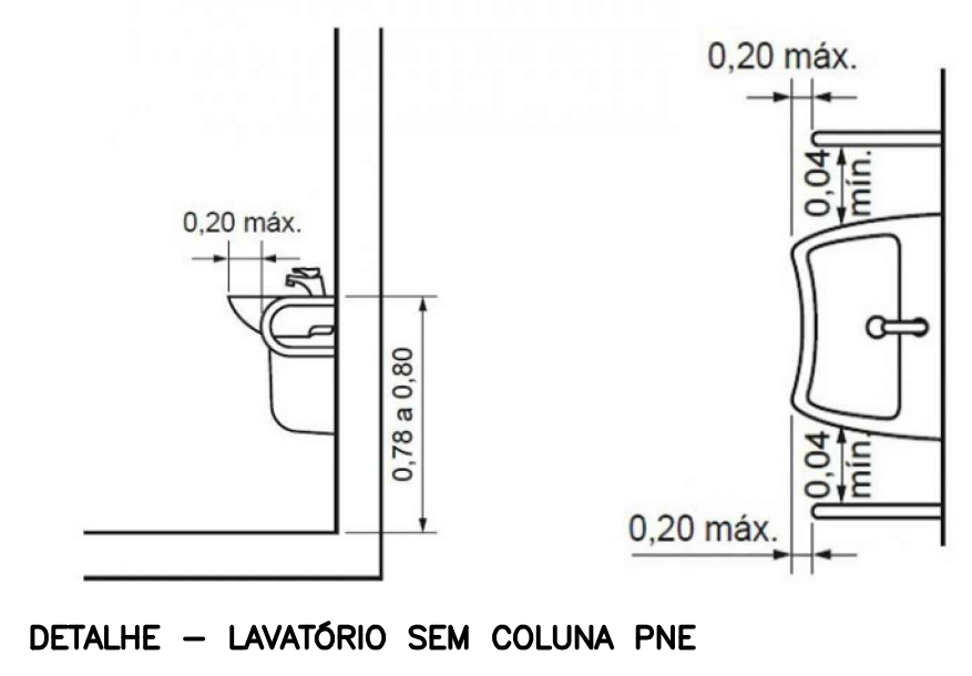
DETALHE - LAVATÓRIO SEM COLUNA PNE
