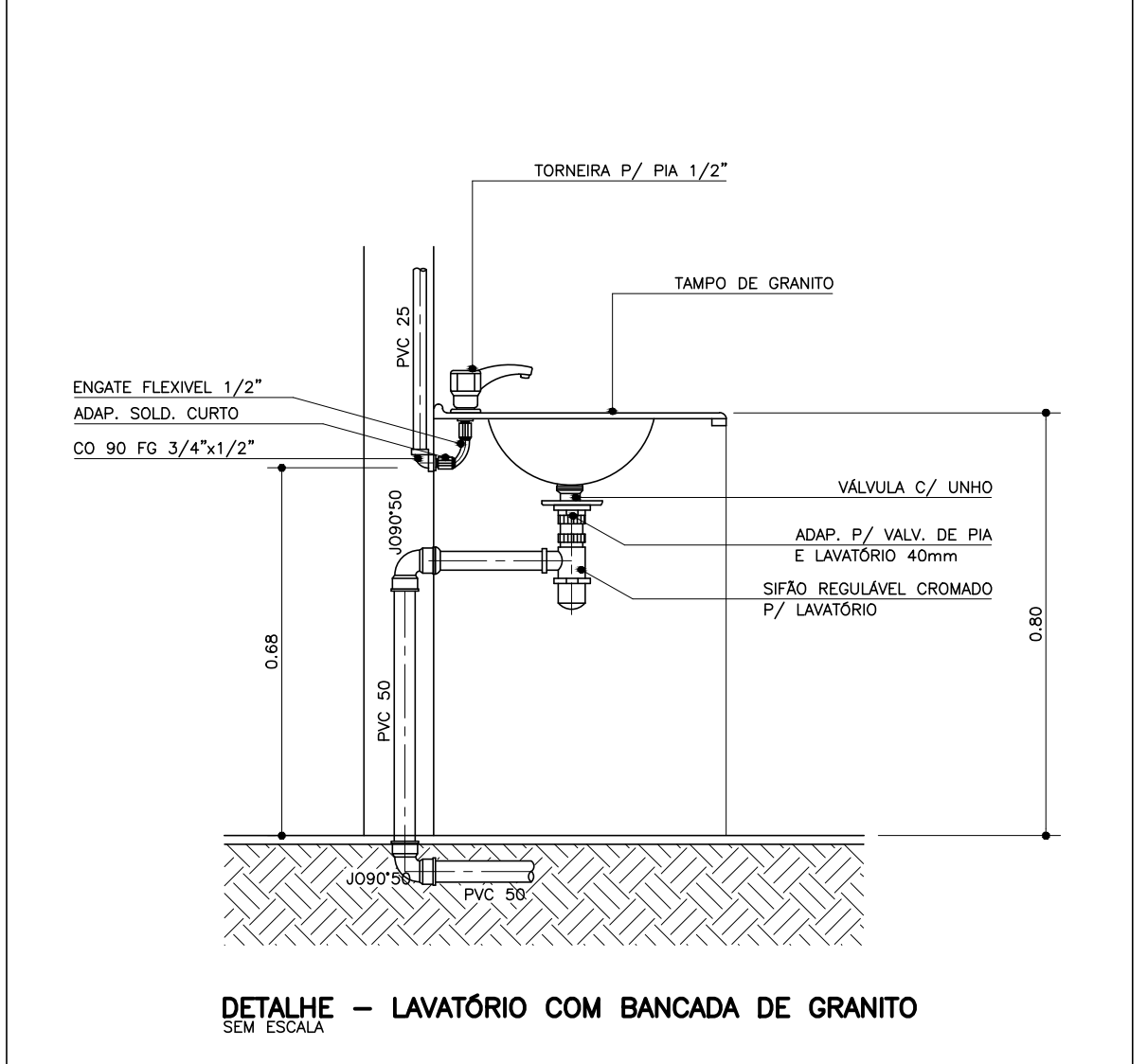
IMAGEM ILUSTRATIVA - DETALHE INSTALAÇÃO REDE DE ESGOTO (LAVATÓRIO COM BANCADA DE GRANITO)
