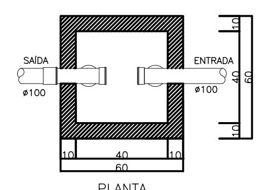
Detalhe da Caixa de Gordura (CG) Sem Esc.
