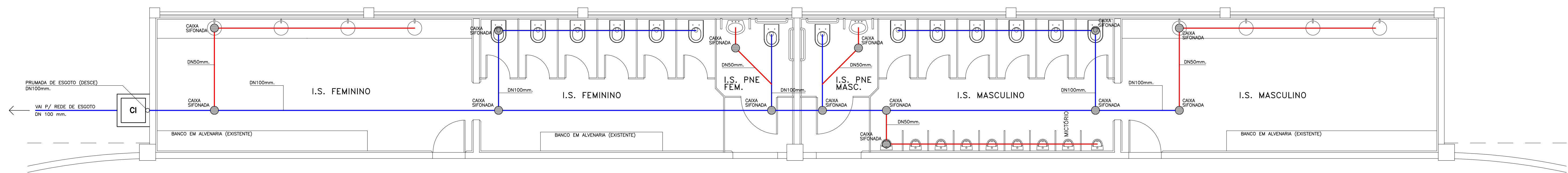
PLANTA - REDE DE ESGOTO ESCALA : 1:50
