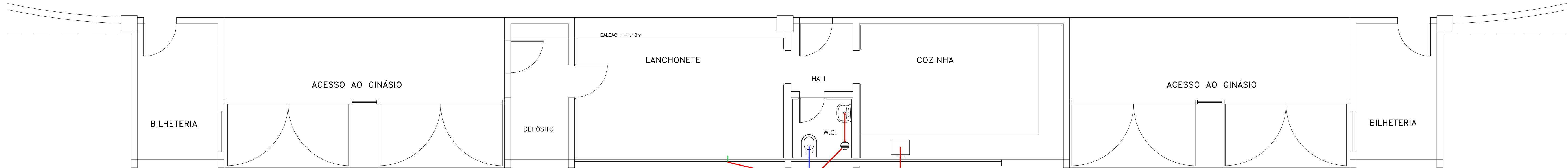
PLANTA - REDE DE ESGOTO ESCALA : 1:50
