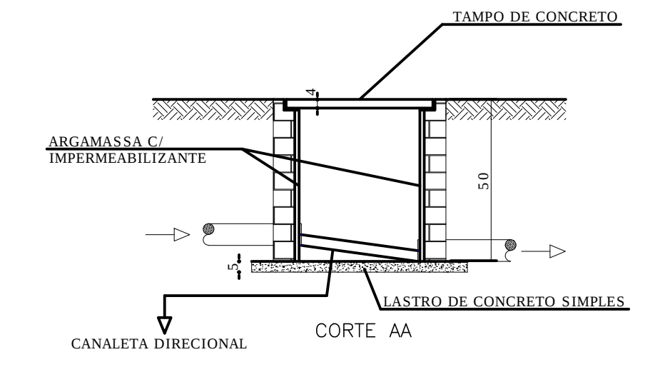
Detalhe da Caixa de Inspeção (CI) Sem Esc.
