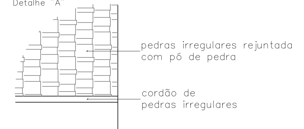
Detalhe "A"
