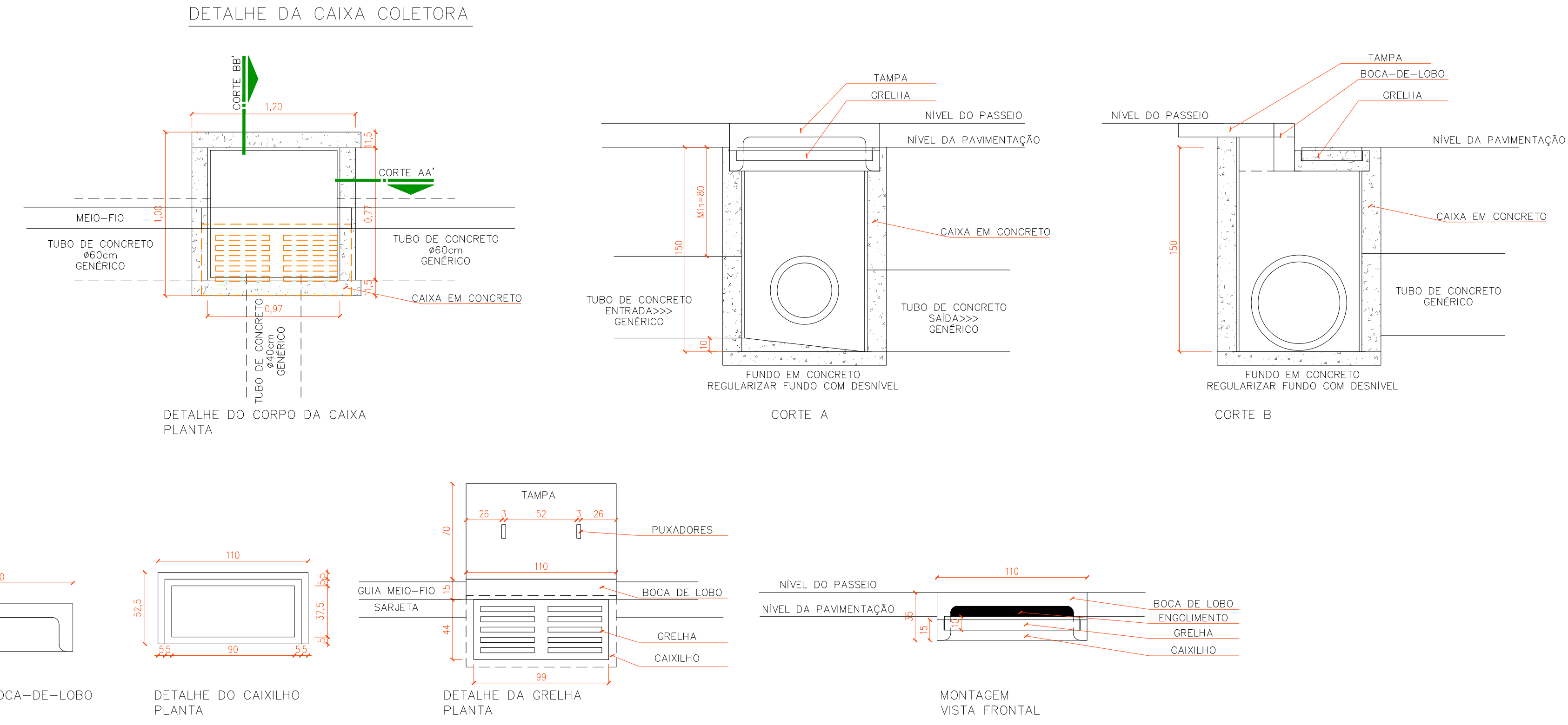
DETALHE DA CAPTAÇÃO ESCALA: 1/25
