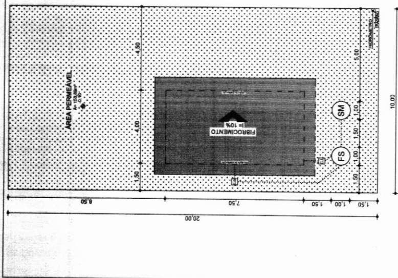
PLANTA DE IMPLANTAÇÃO ESC.: 1/100
