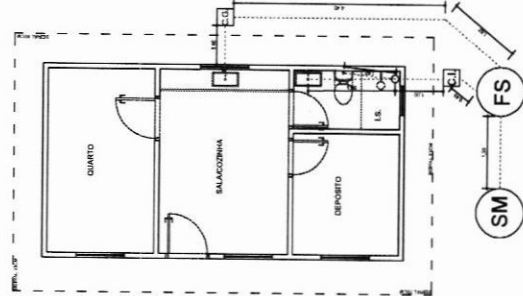
PLANTA BAIXA - HIDROSSANITÁRIO ESC.: 1/75
