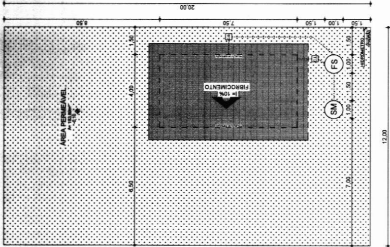
PLANTA DE IMPLANTAÇÃO ESC.: 1/100
