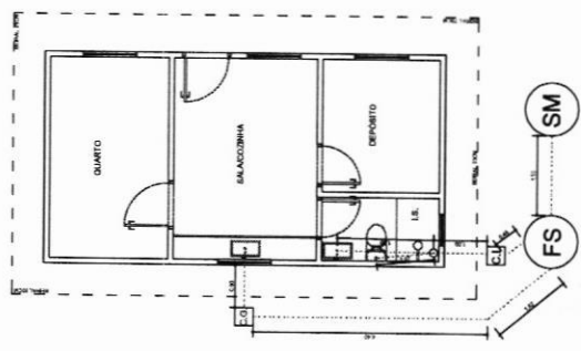
PLANTA BAIXA - HIDROSSANITÁRIO ESC.: 1/75
