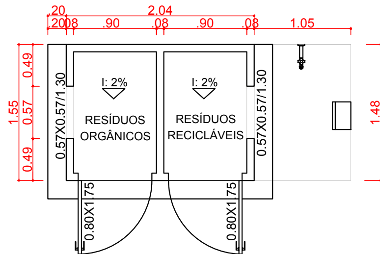
Planta Baixa
