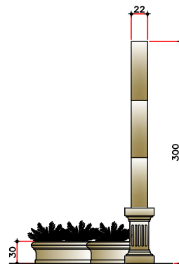
ELEVAÇÃO LATERAL
