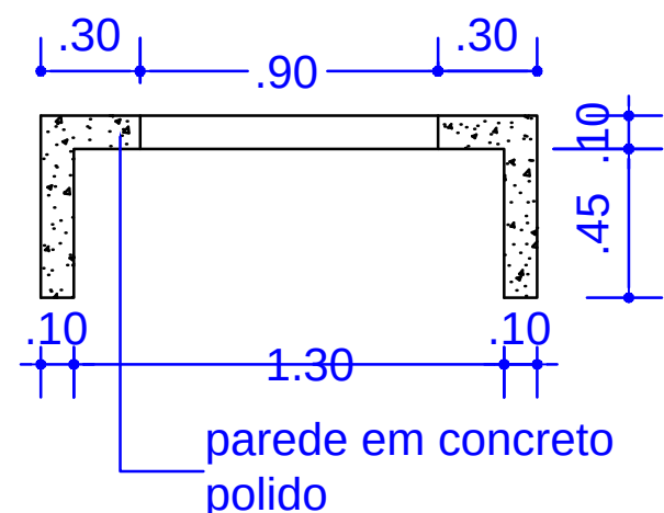
CORTE AA - BANCO
