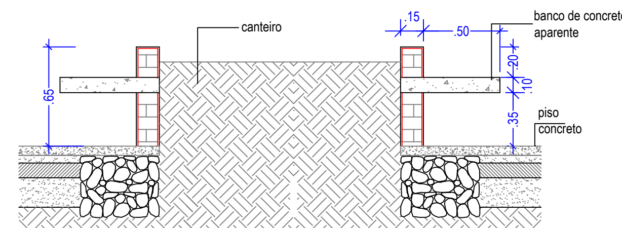
CORTE BB - BANCO CONCRETO
