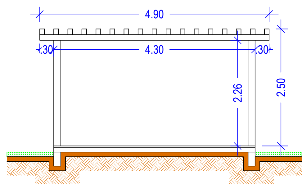
CORTE AA - PERGOLADO
