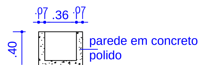
CORTE AA - FLOREIRA
