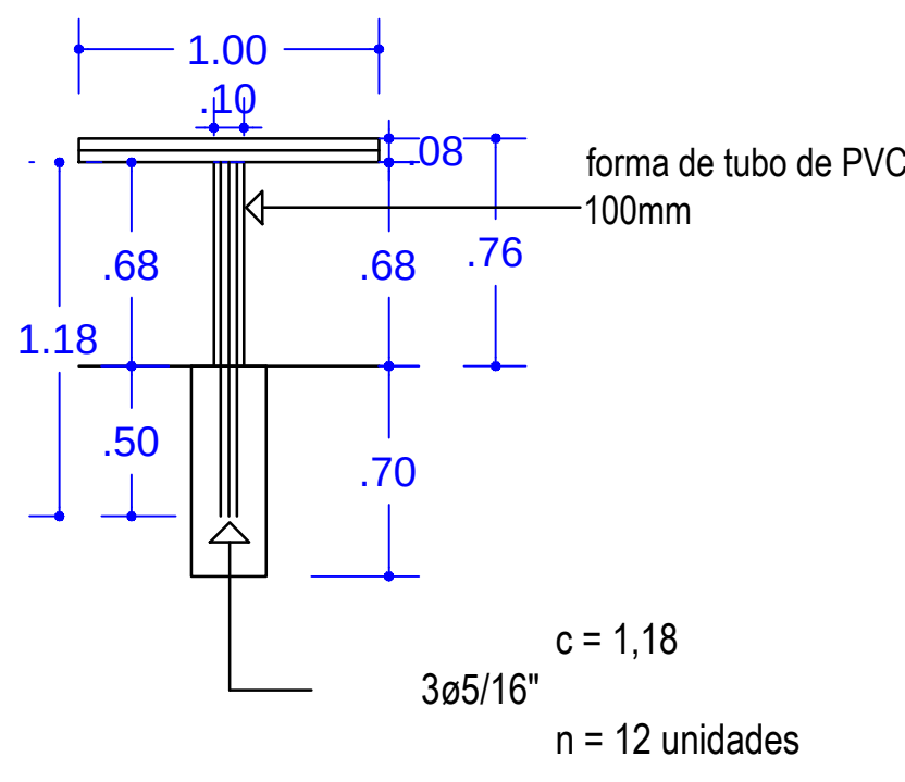
CORTE TRANSVERSAL
