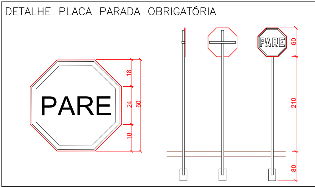
DETALHE - SINALIZAÇÃO VERTICAL SEM ESCALA
