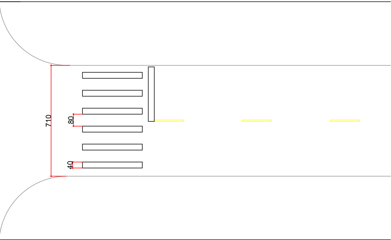
DETALHE - SINALIZAÇÃO HORIZONTAL SEM ESCALA
