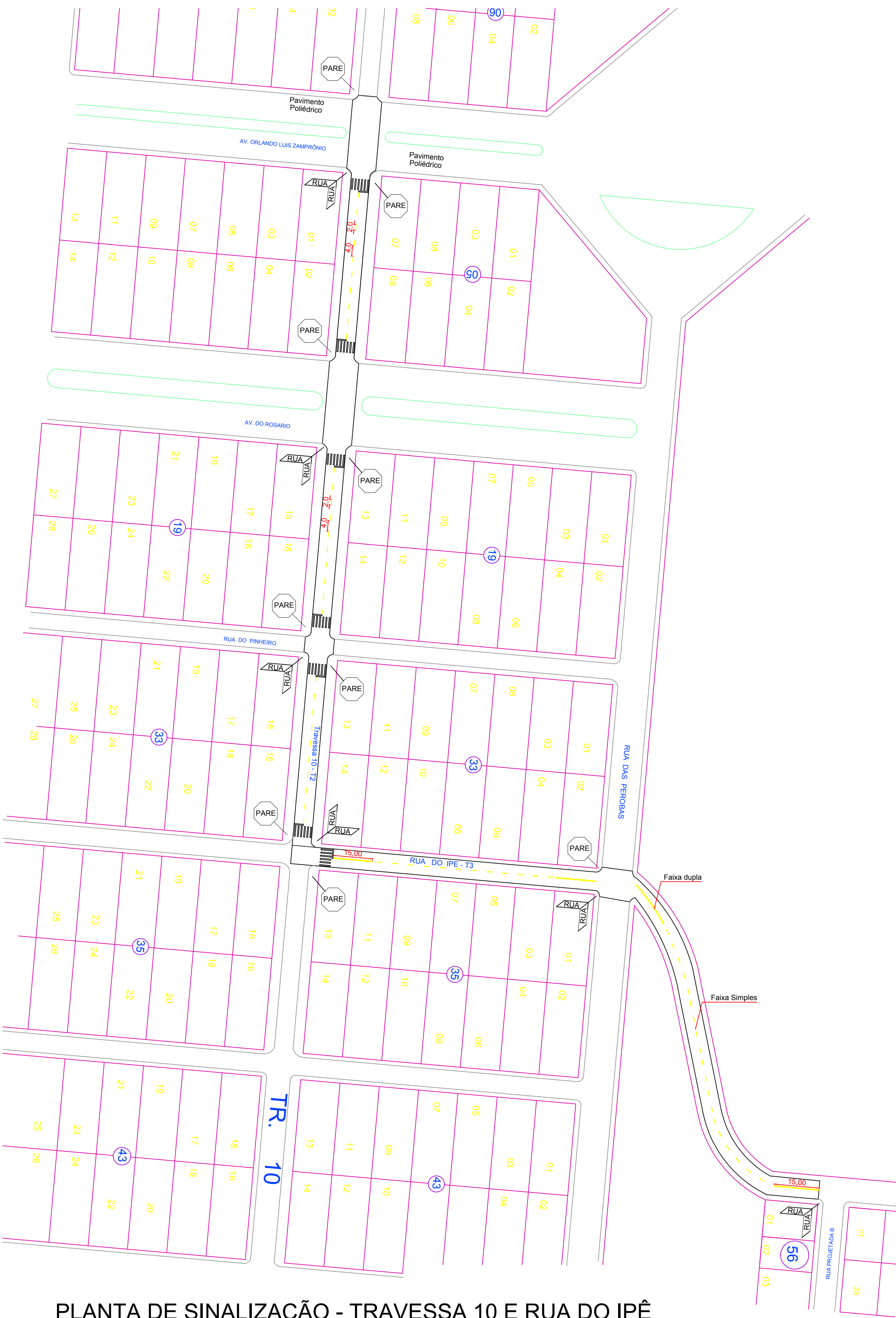
PLANTA DE SINALIZAÇÃO - TRAVESSA 10 E RUA DO IPÊ ESCALA: 1/1000
