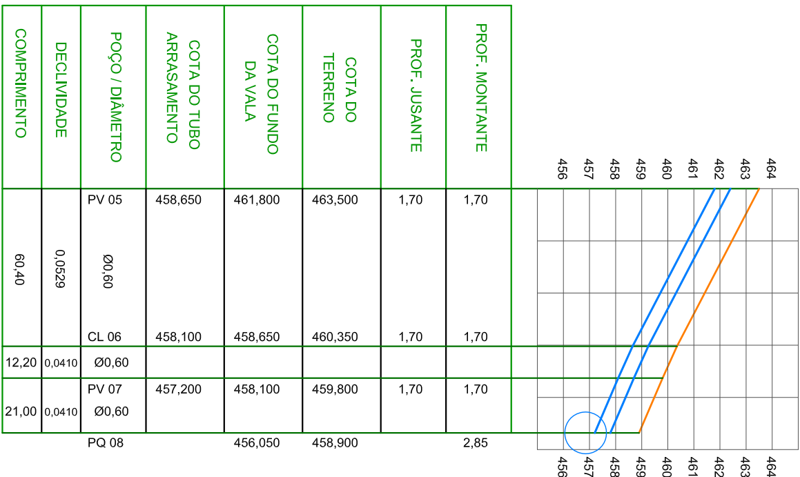
PERFIL DA RUA MOISÉS CAROLINO FILHO ESCALA VERTICAL 1:200 ESCALA HORIZONT 1:2.000
