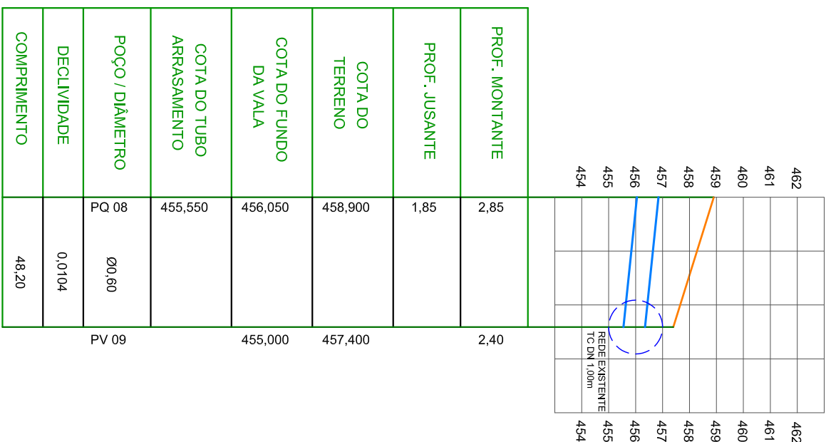
PERFIL DO EMISSÁRIO ESCALA VERTICAL 1:200 ESCALA HORIZONT 1:2.000
