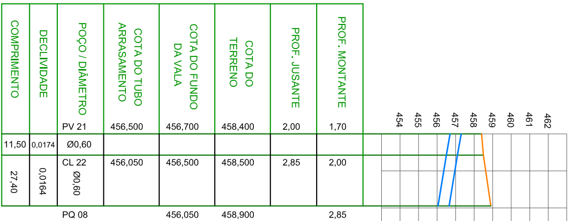
PERFIL DA RUA MOISÉS CAROLINO FILHO ESCALA VERTICAL 1:200 ESCALA HORIZONT 1:2.000
