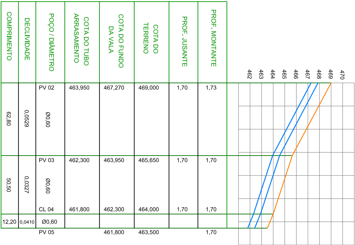
PERFIL DA RUA TEODORINA CÂNDIDA BATISTA ESCALA VERTICAL 1:200 ESCALA HORIZONT 1:2.000
