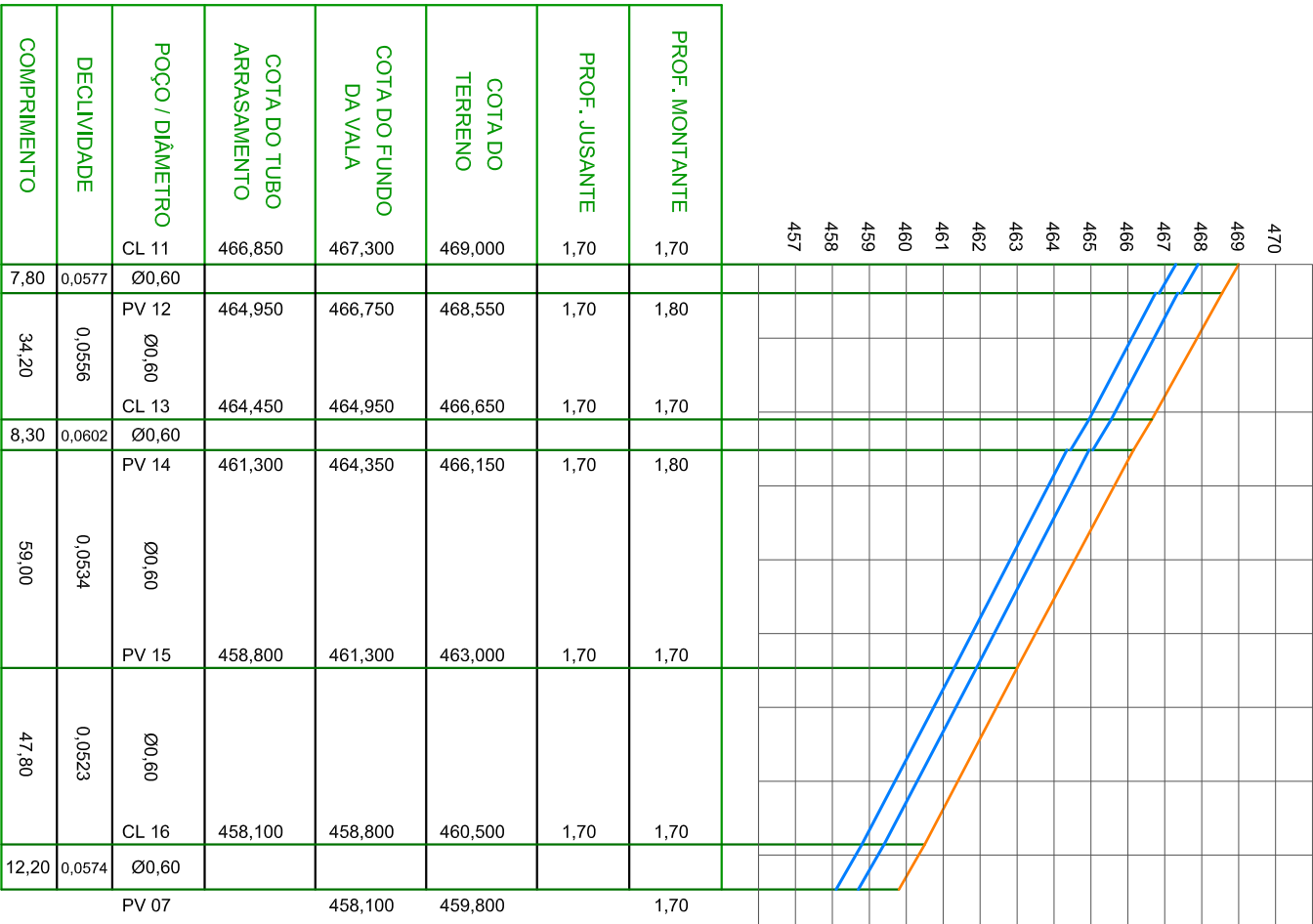
PERFIL DA RUA ILDEBRANDO SERTORI ESCALA VERTICAL 1:200 ESCALA HORIZONT 1:2.000
