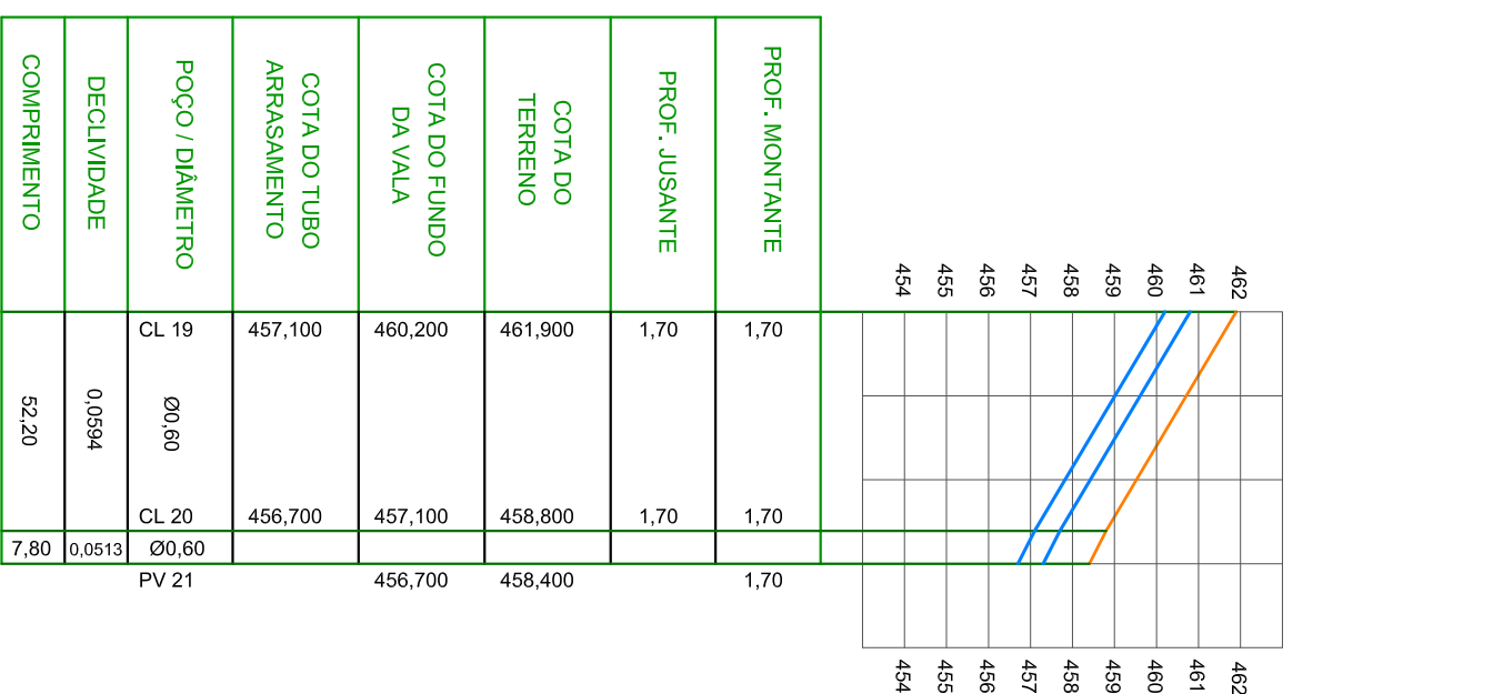
PERFIL DA RUA CAMPOS ELÍSEOS ESCALA VERTICAL 1:200 ESCALA HORIZONT 1:2.000
