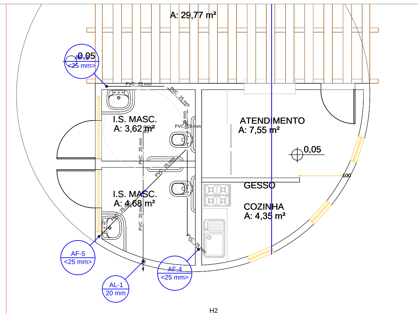
PLANTA BAIXA - COBERTURA ESCALA 1/50
