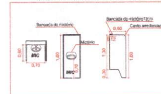
DETALHE DIVISÓRIAS DOS MICTÓRIOS EM GRANITO
