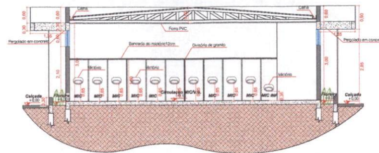
CORTE A-A 1:2
