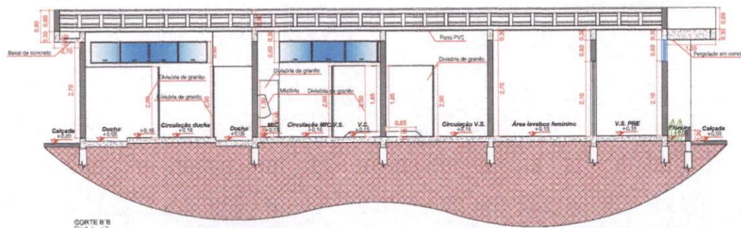
CORTE B-B 1:2
