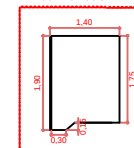
DETALHE DIVISÓRIAS DOS SANITÁRIOS EM GRANITO
