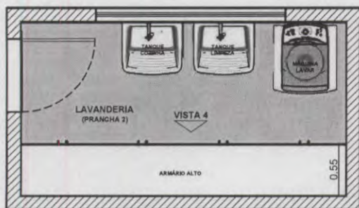
PLANTA BAIXA LAVANDERIA (PRANCHA 2)
