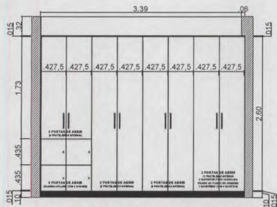
VISTA 4 - EXTERNO ARMÁRIO LAVANDERIA (PRANCHA 2)
