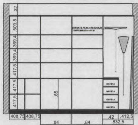
VISTA 4 - INTERNO ARMÁRIO LAVANDERIA (PRANCHA 2)
