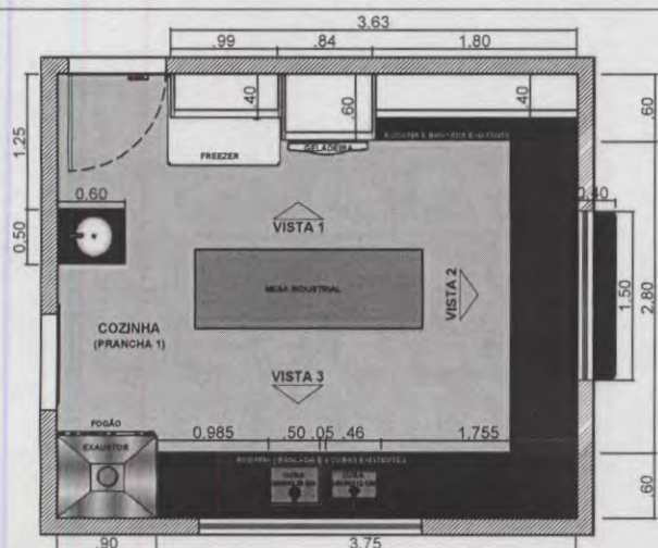
PLANTA BAIXA COZINHA PORTO DOS SANTOS (PRANCHA 1)
