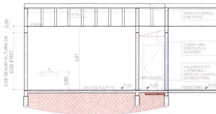
CORTE CC'
