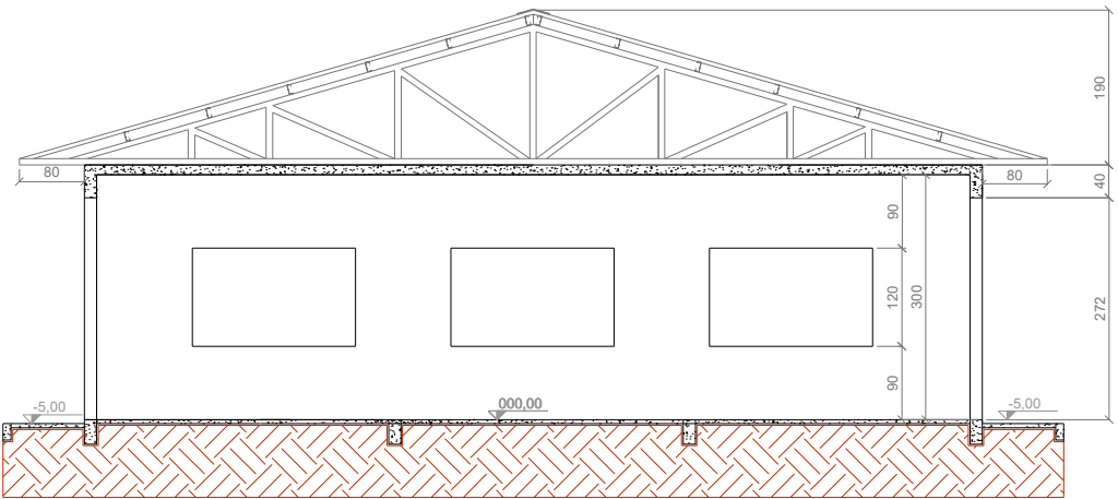
CORTE A-B Esc:.....1/50
