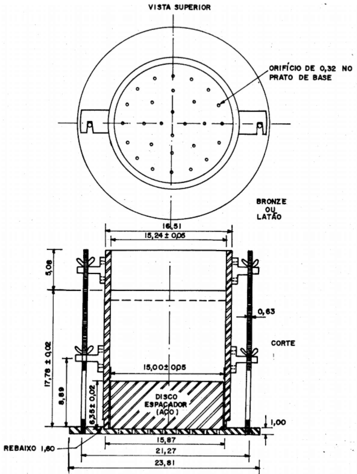
Figura 1 – Molde cilíndrico, cilindro complementar e base metálica
