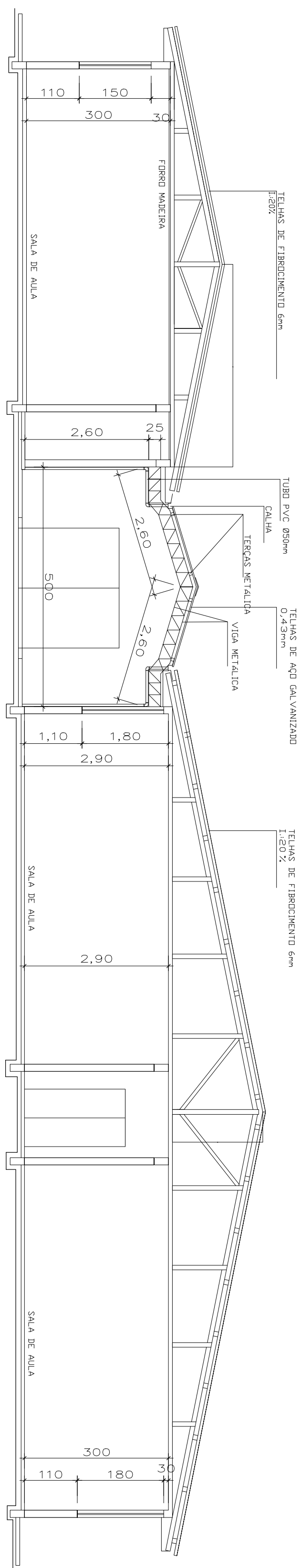
CORTE AA - ESC. 1:75
