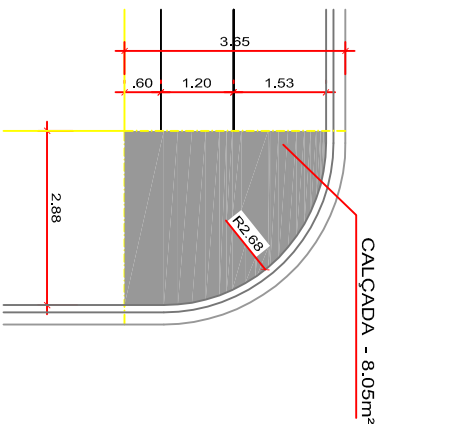
DETALHE - SETOR S02
