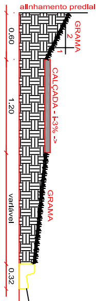
DETALHE PASSEIO COM DESNIVEL
