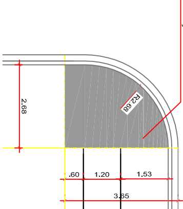
DETALHE - SETOR S03
