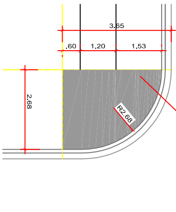
DETALHE - SETOR S04
