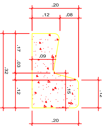
DETALHE MEIO-FIO/SARJETEA
