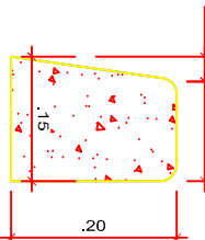
DETALHE MEIO-FIO
