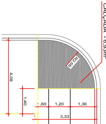
DETALHE - SETOR S05
