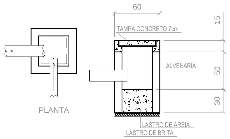
DETALHE DA CAIXA DE AREIA A Esc: ..... 1/25
