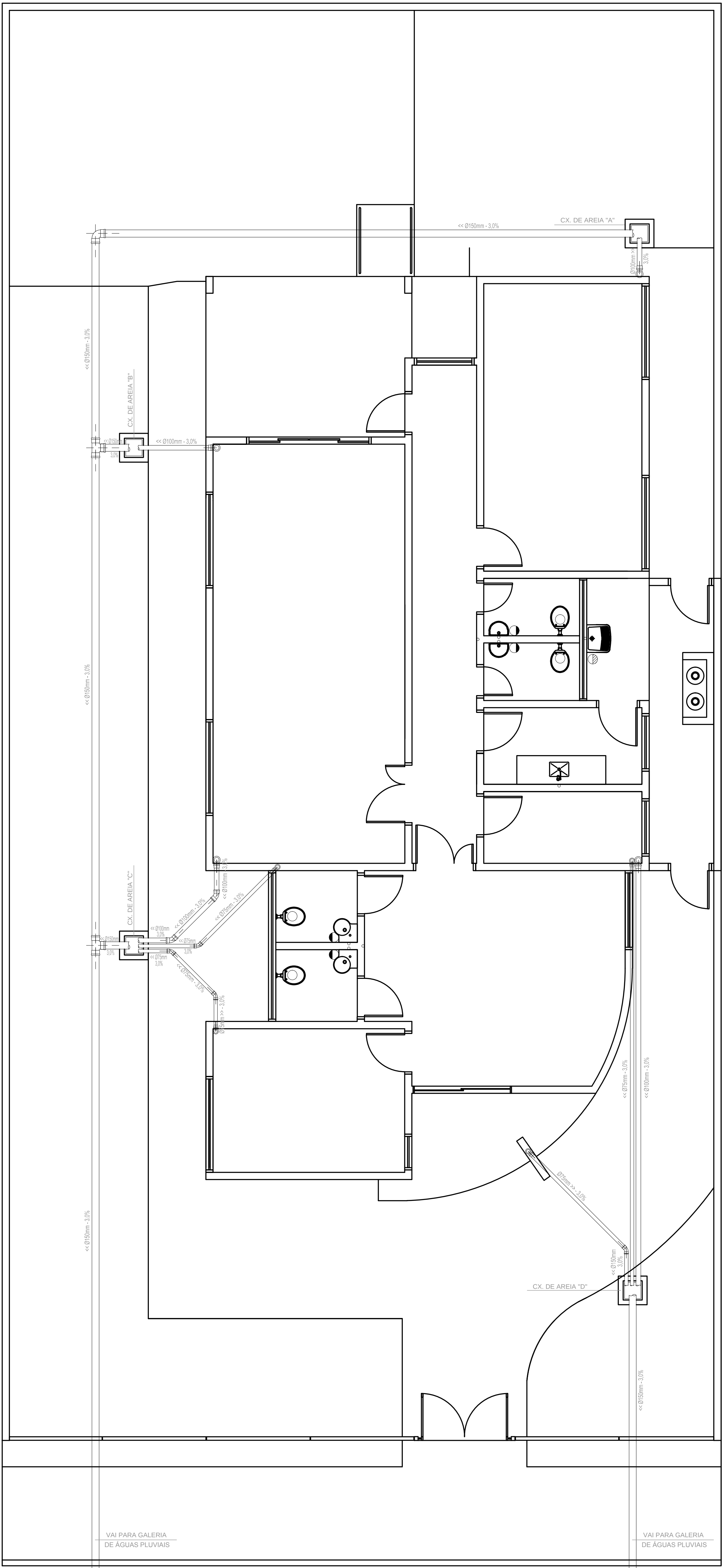
PLANTA DE LOCAÇÃO DE TUBULAÇÕES DE ÁGUAS PLUVIAIS Esc:.....1/50
