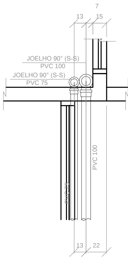
DETALHE DE TUB. DE ÁGUAS PLUVIAIS "E" Esc:.....1/25
