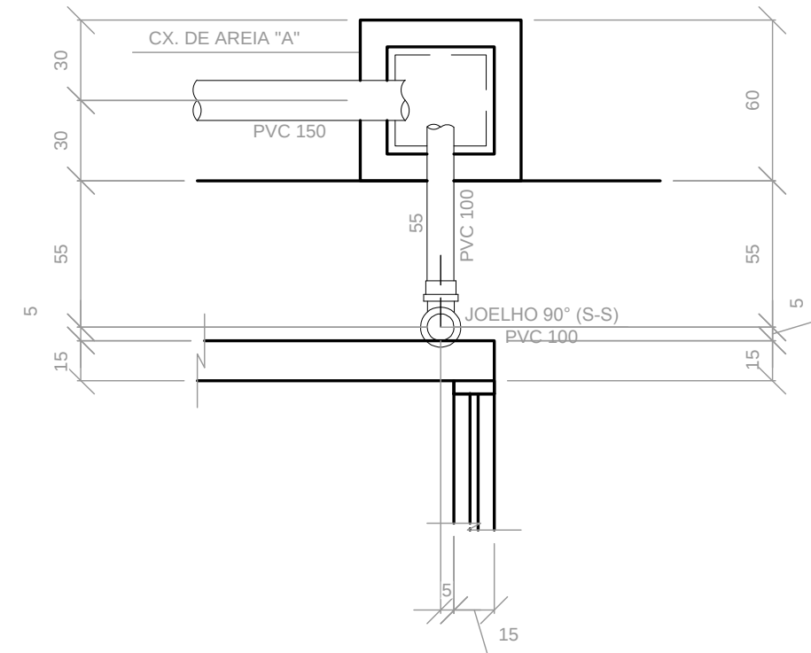
DETALHE DE TUB. DE ÁGUAS PLUVIAIS "A" Esc:.....1/25
