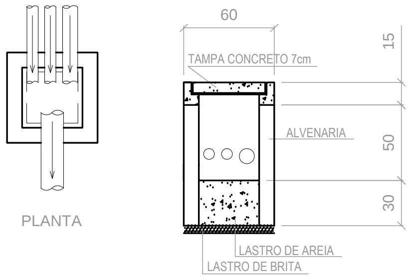
DETALHE DA CAIXA DE AREIA D Esc: ..... 1/25
