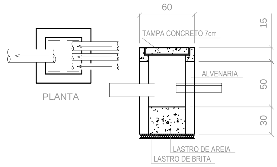
DETALHE DA CAIXA DE AREIA C Esc: ..... 1/25
