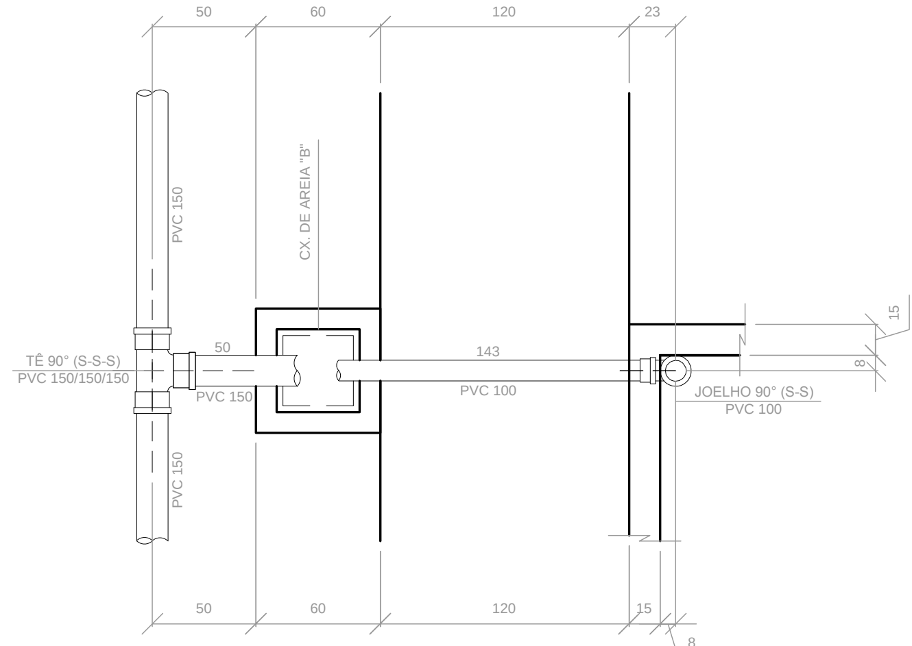
DETALHE DE TUB. DE ÁGUAS PLUVIAIS "B" Esc:.....1/25
