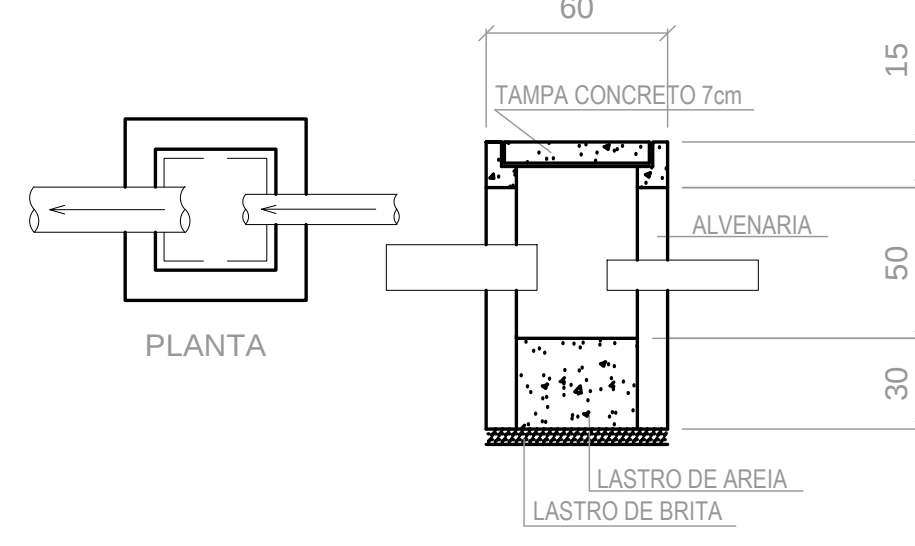
DETALHE DA CAIXA DE AREIA B Esc: ..... 1/25
