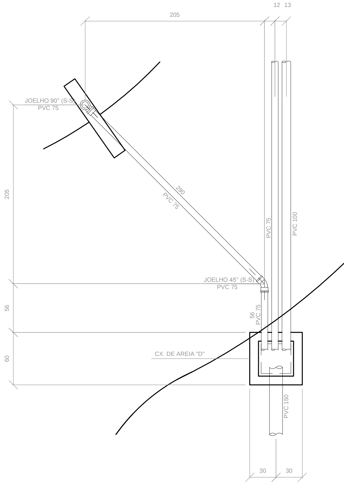
DETALHE DE TUB. DE ÁGUAS PLUVIAIS "D" Esc:.....1/25
