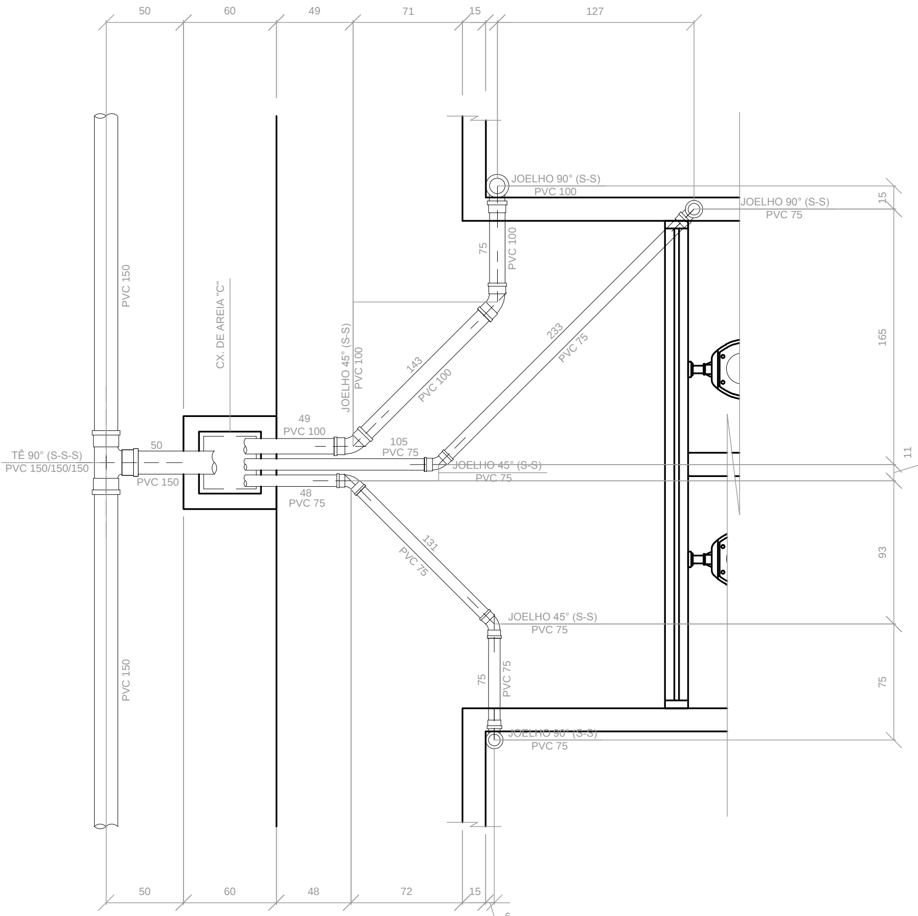
DETALHE DE TUB. DE ÁGUAS PLUVIAIS "C" Esc:.....1/25
