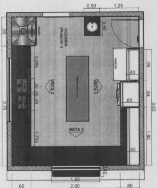
PLANTA BAIXA COZINHA PORTO DOS SANTOS (PRANCHA 1)
