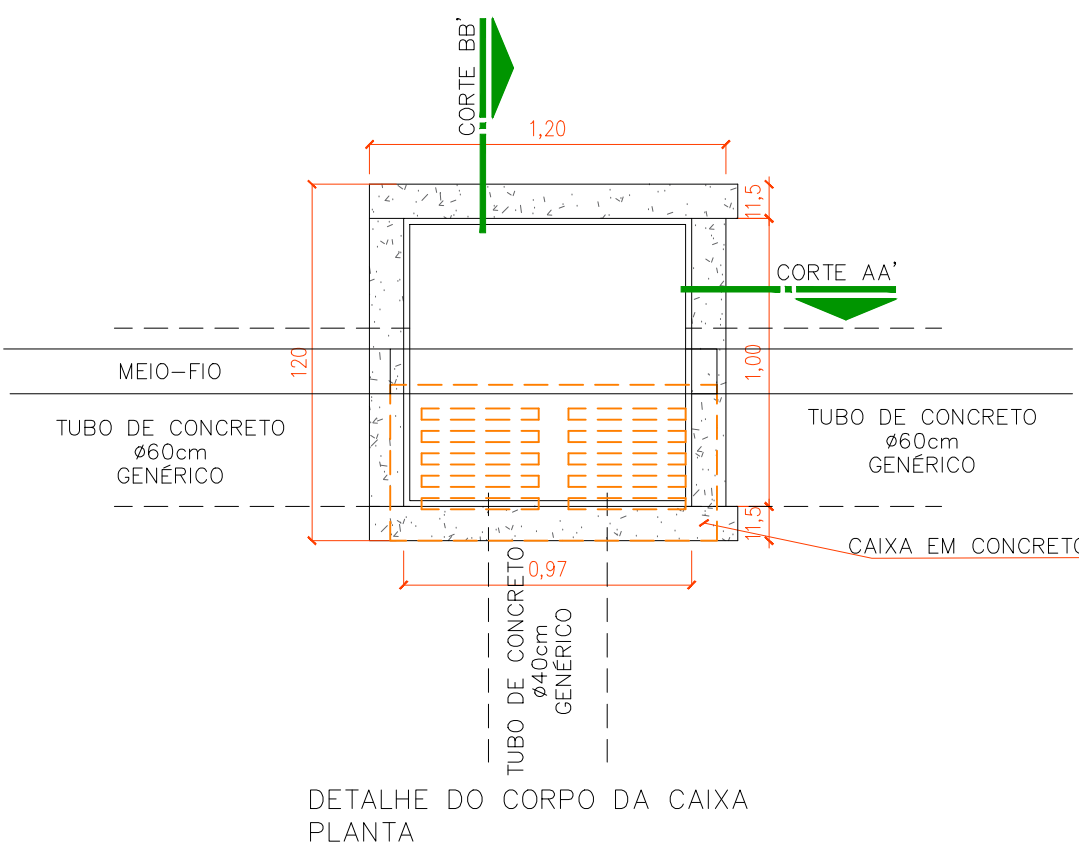
DETALHE DA CAIXA COLETORA
