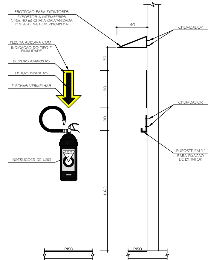
Det. Fixação e Sinalização Parede Esc. 1:20
