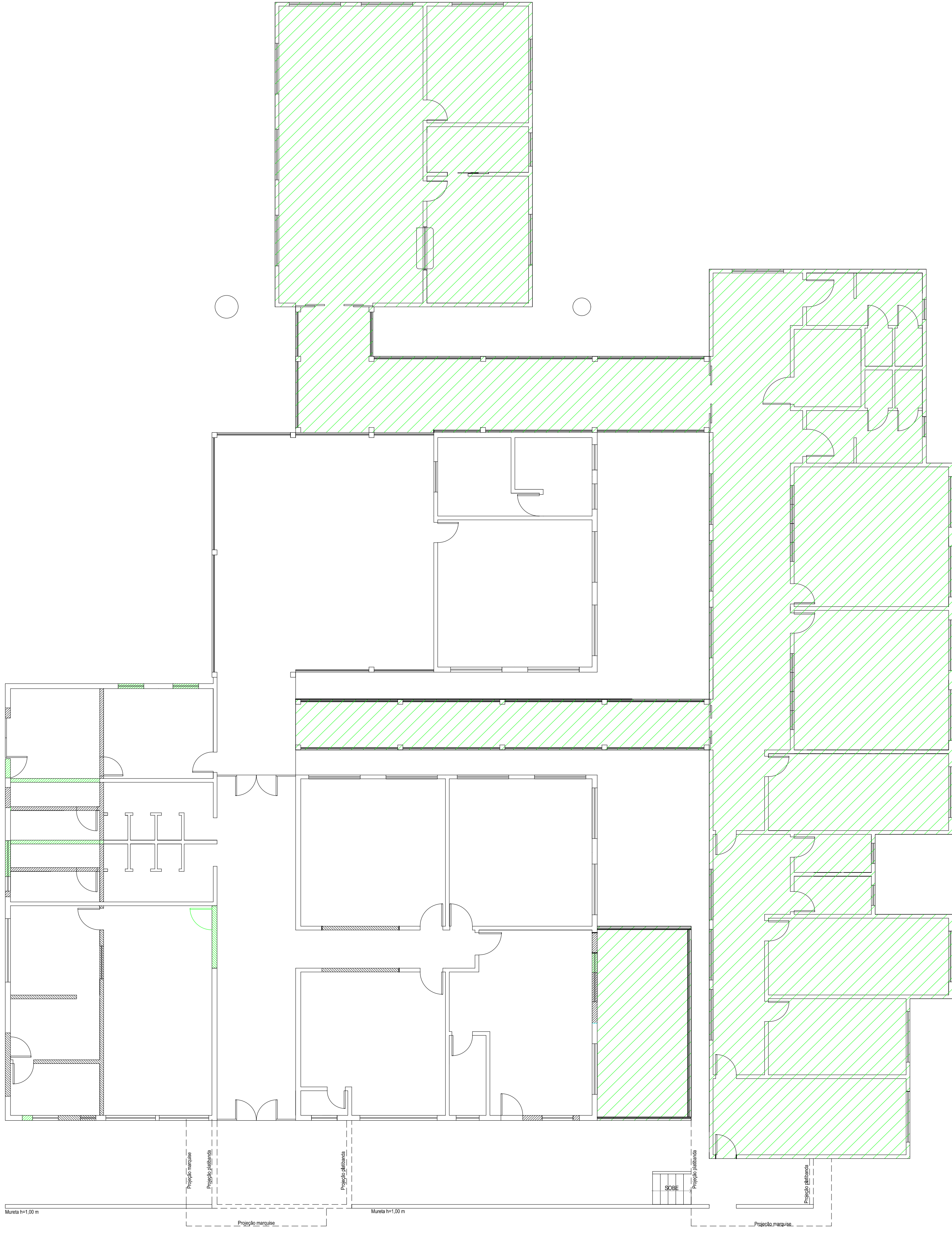
PLANTA BAIXA CONSTRUIR/ DEMOLIR Esc.: 1:100
