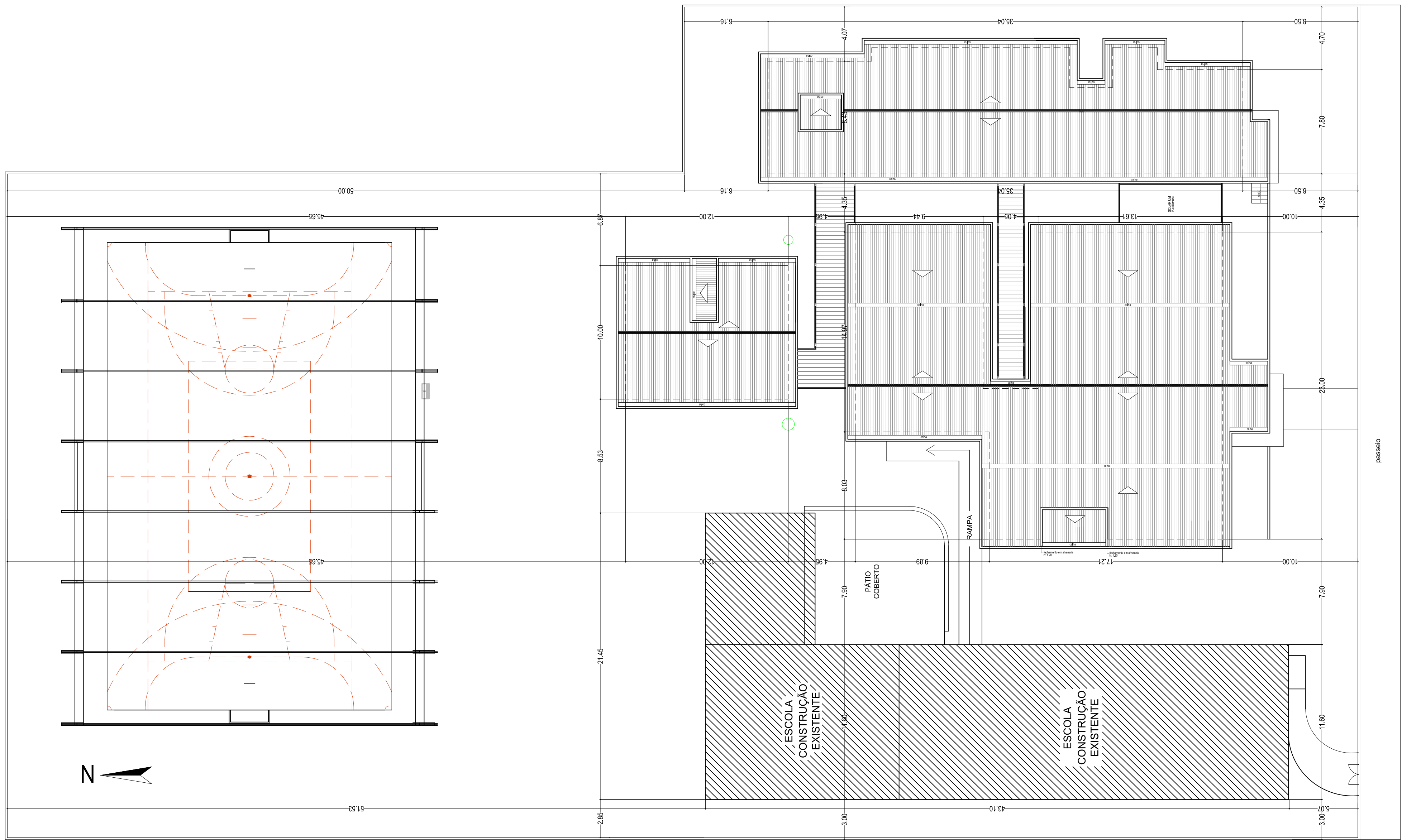
PLANTA DE COBERTURA/IMPLANTAÇÃO Esc.: 1:200
