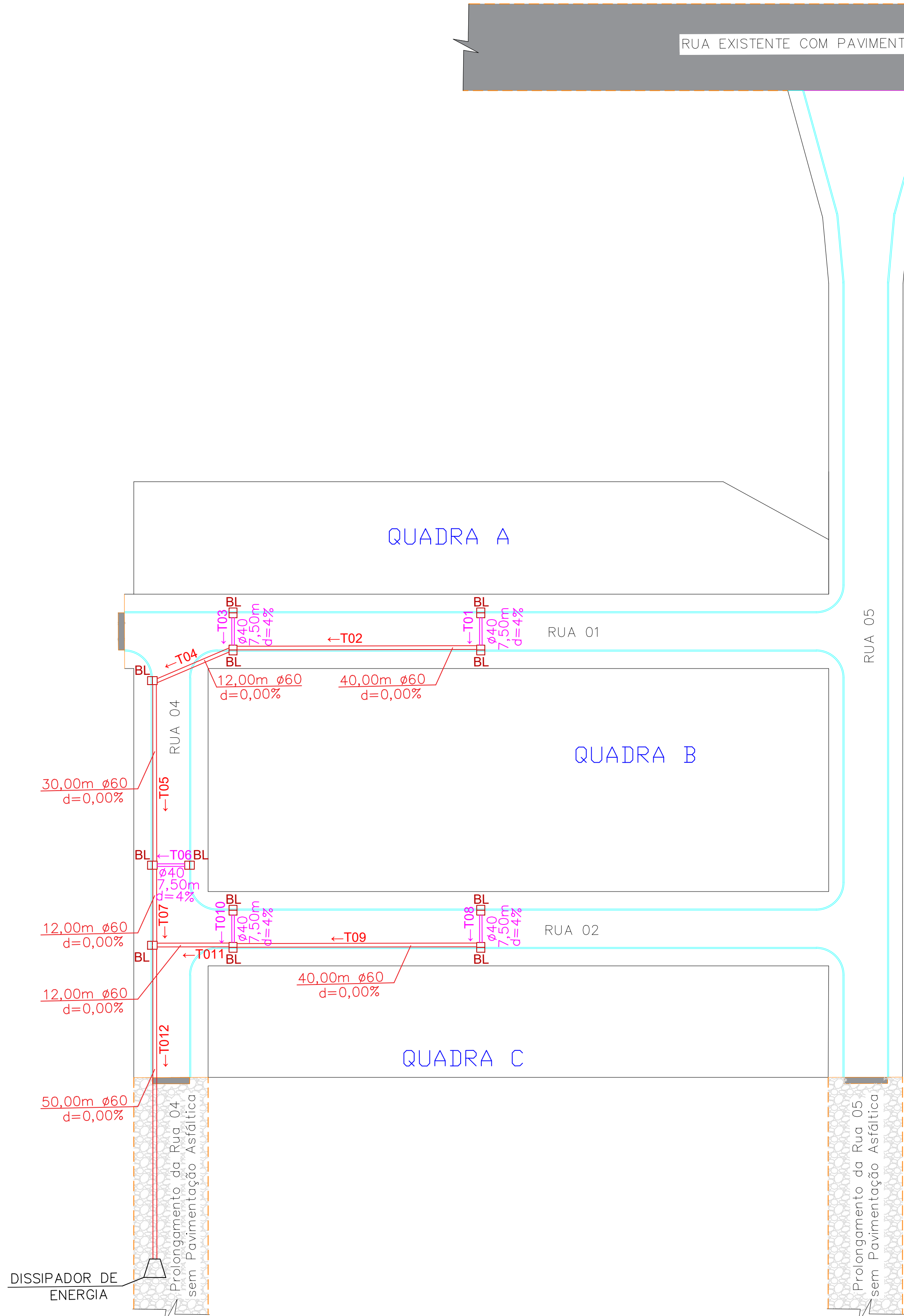
PLANTA BAIXA DRENAGEM ESCALA: 1/500
