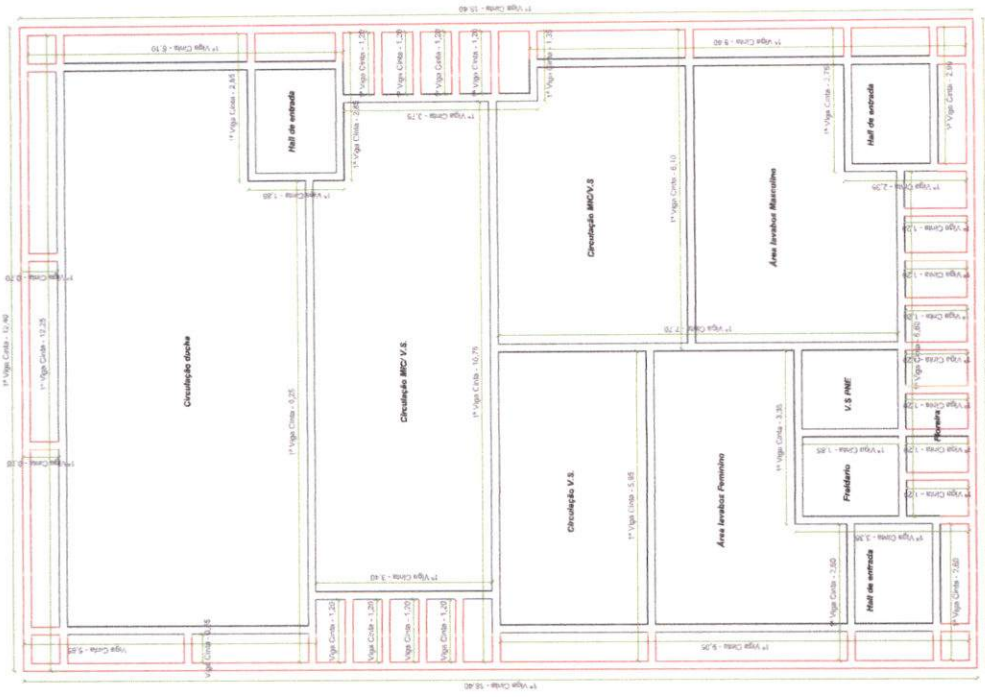
PLANTA BAIXA - 1ª VIGAS CINTAS
