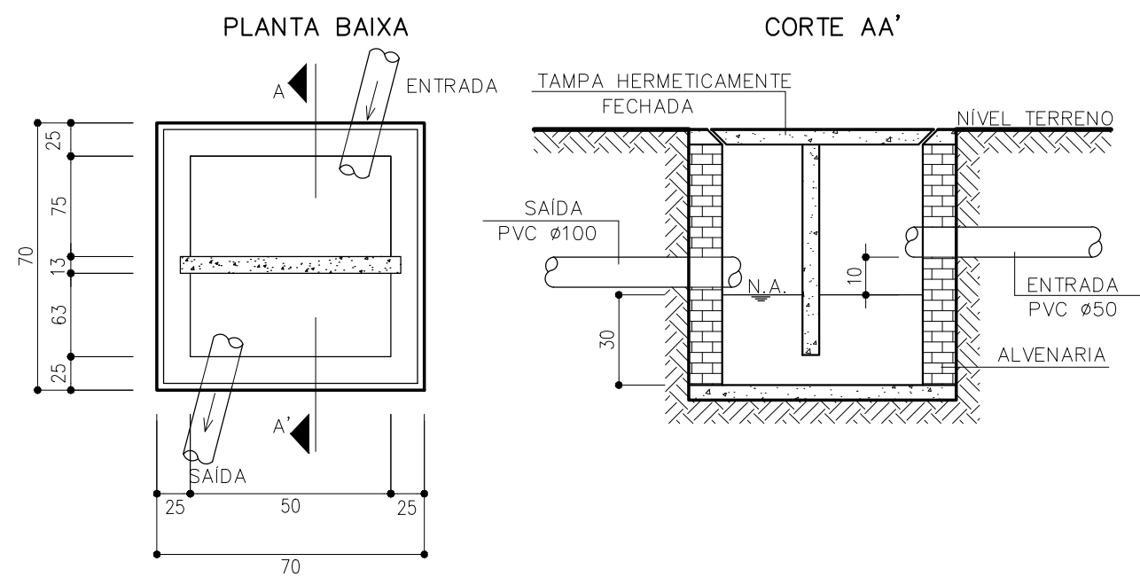
PLANTA BAIXA RESERVATÓRIO COM SUAS LIGAÇÕES SEM ESCALA
