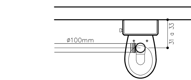
DISTÂNCIA DO PONTO DE ESGOTO DO VASO SANITÁRIO ESCALA: 1/25
