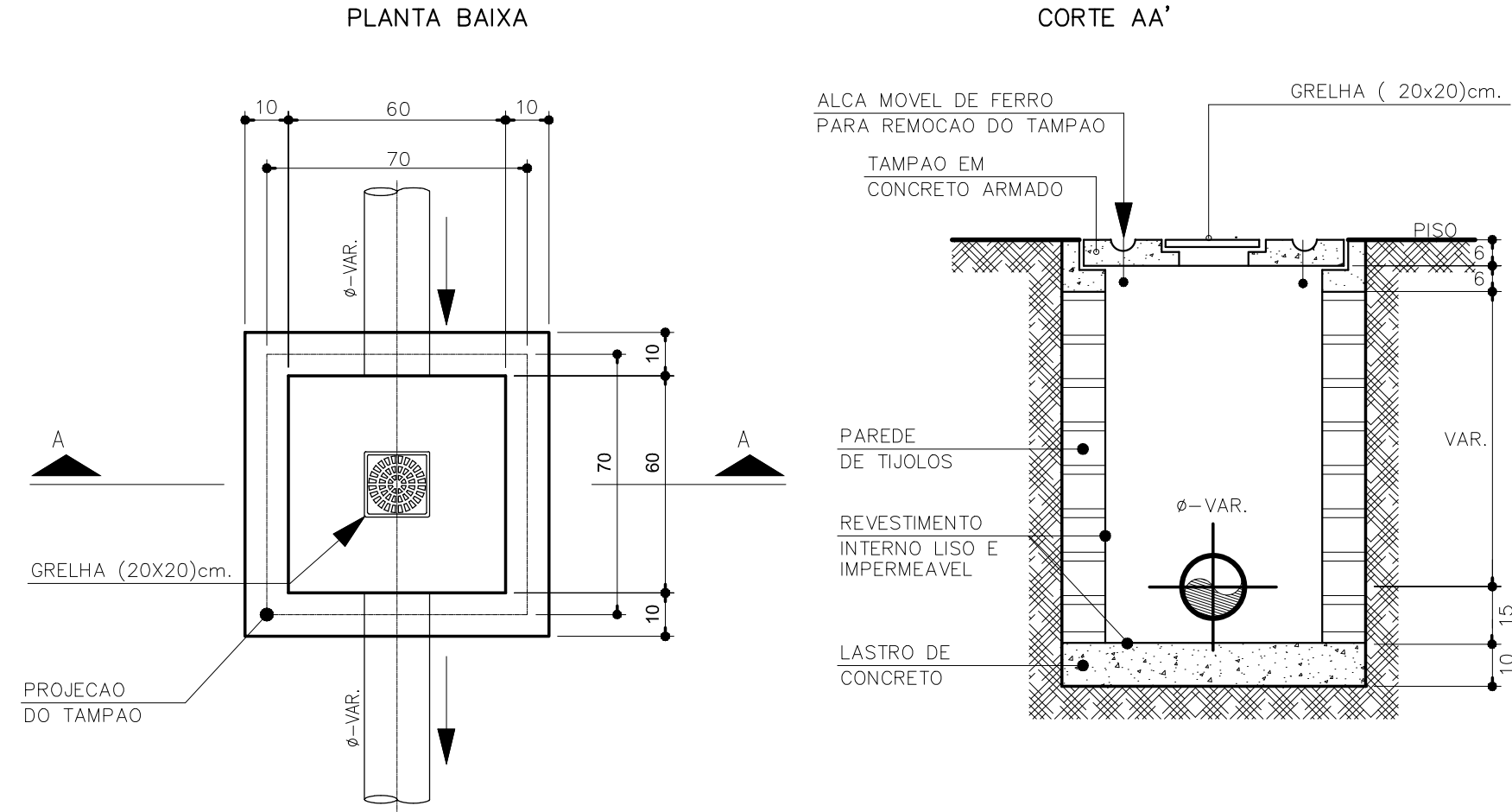
DET. CX. DE CAPTACAO SEM ESCALA
