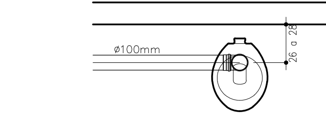
DISTÂNCIA DO PONTO DE ESGOTO DO VASO SANITÁRIO ESCALA: 1/25
