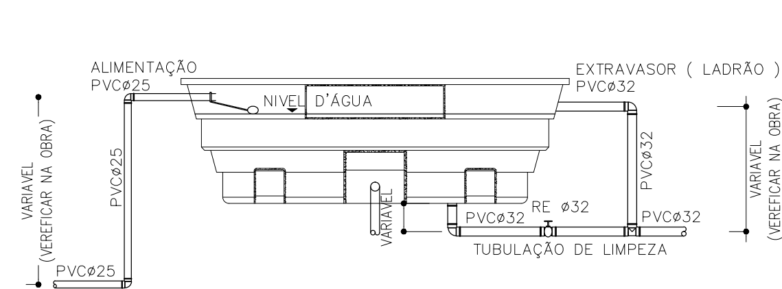
VISTA LATERAL I RESERVATÓRIO COM SUAS LIGAÇÕES SEM ESCALA
