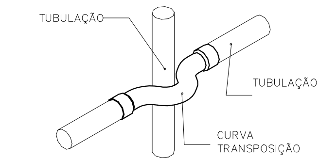
DETALHES DESVIO DE TUBULAÇÃO ESCALA: 1/25
