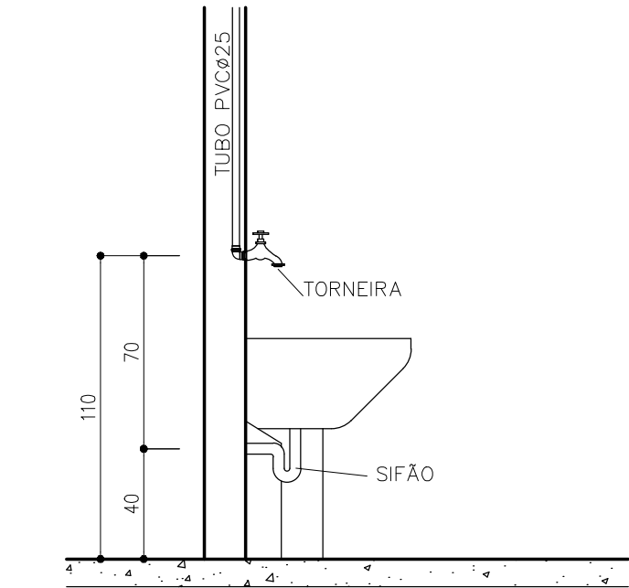
DET. GENÉRICO PARA TANQUE ESCALA: 1/25
