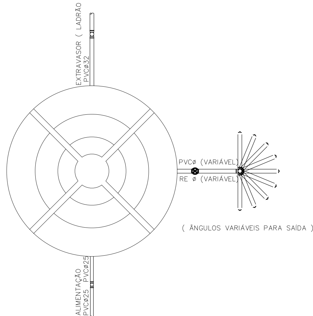
PLANTA BAIXA RESERVATÓRIO COM SUAS LIGAÇÕES SEM ESCALA
