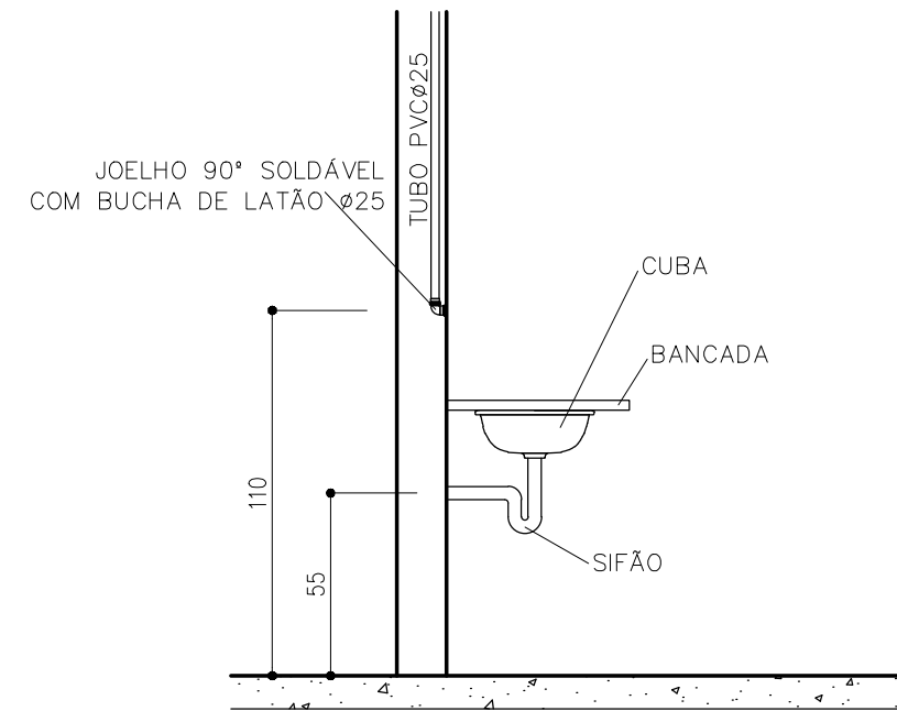
DET. GENÉRICO PARA PIA SEM ESCALA
