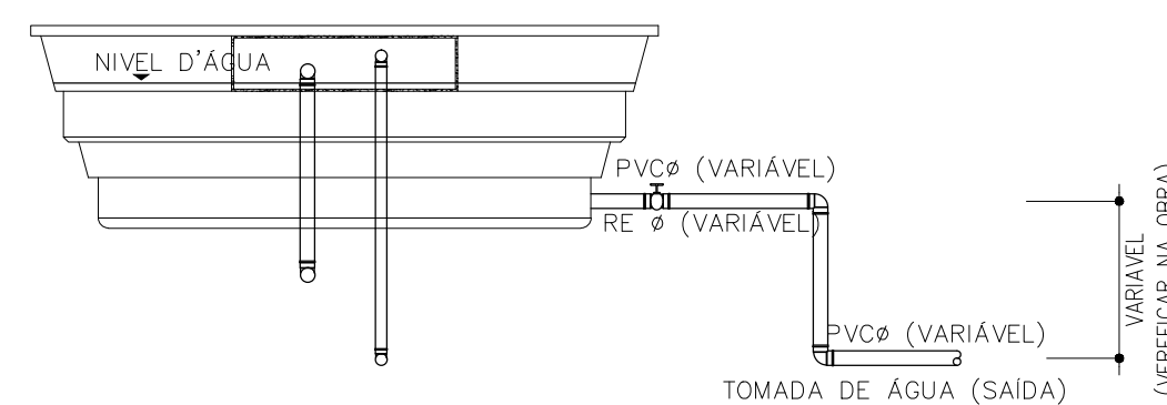
VISTA LATERAL II RESERVATÓRIO COM SUAS LIGAÇÕES SEM ESCALA
