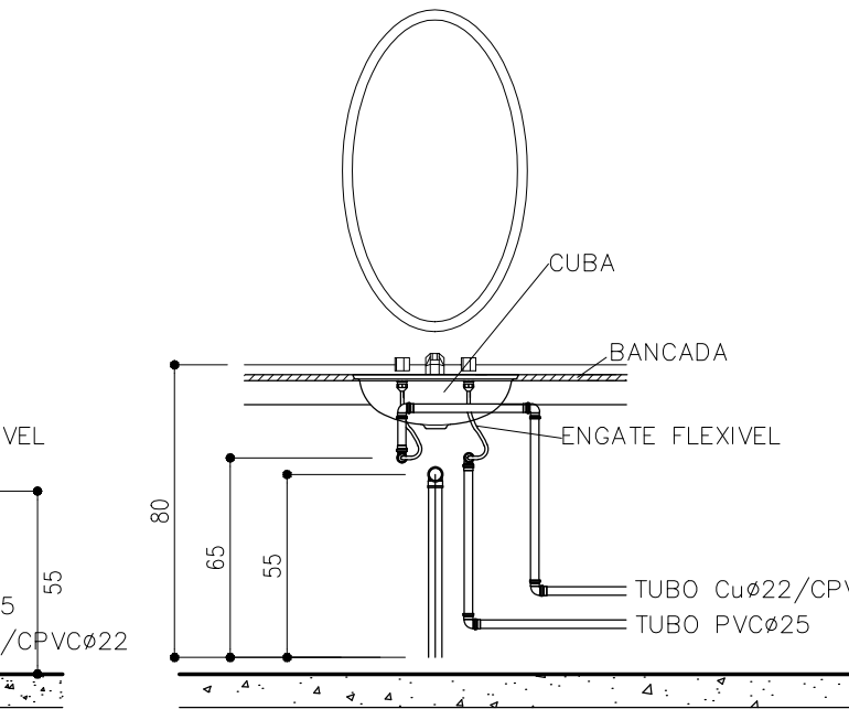
DET. GENÉRICO PARA LAVATÓRIO DE BANCADA ESCALA: 1/25
