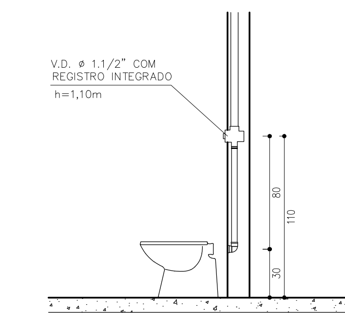
DETALHE VÁLVULA HIDRA ESCALA: 1/25
