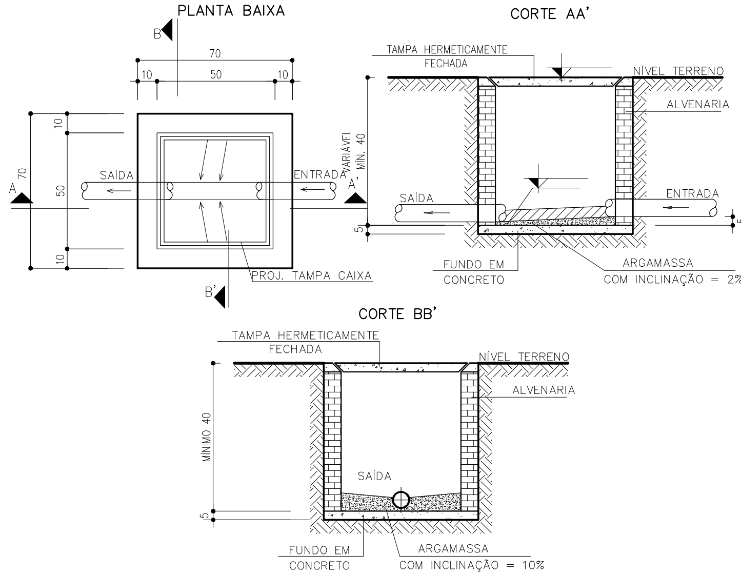
DET. CAIXA DE INSPEÇÃO SEM ESCALA
