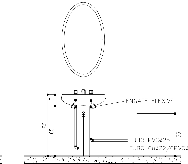
DET. GENÉRICO PARA LAVATÓRIO DE COLUNA ESCALA: 1/25
