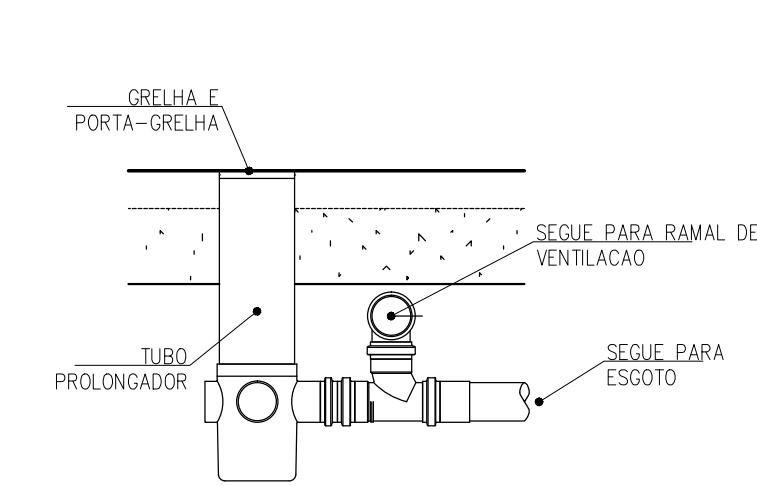
VISTA TÍPICA DE VENTILAÇÃO DE CAIXA SIFONADA ESCALA: 1/25
