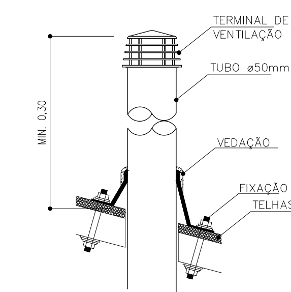
DET. TUBO DE VENTILAÇÃO ESCALA: 1/25
