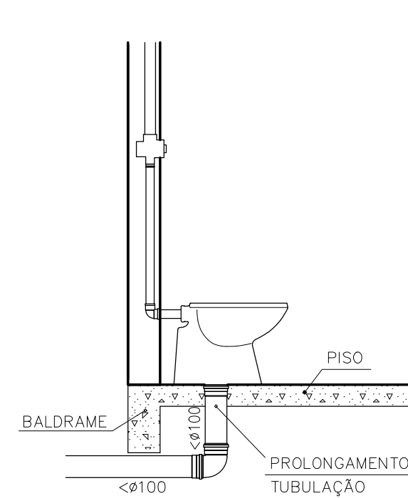
DETALHE SAÍDA ESGOTO TERREO ESCALA: 1/25
