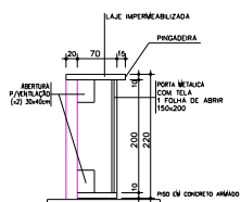
Corte AB ESCALA 1:50
