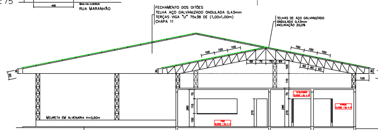
CORTE AB - ESCALA 1:100
