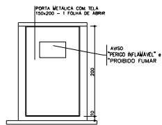
Elevação ESCALA 1:50
