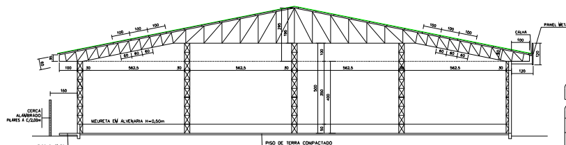
CORTE CD - ESCALA 1:100
