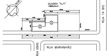
IMPLANTAÇÃO - ESCALA 1/1000
