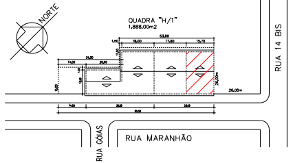
IMPLANTAÇÃO – ESCALA 1/1000
