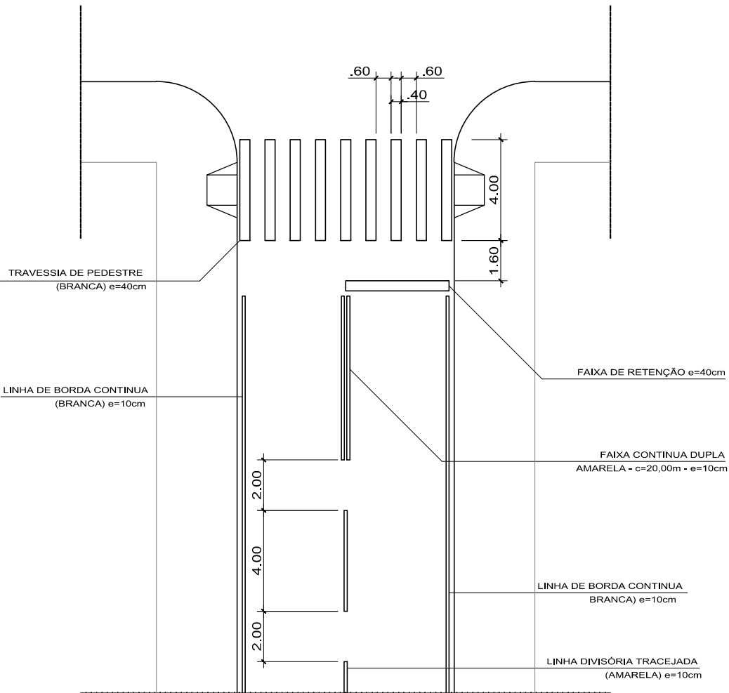
DETALHE SINALIZAÇÃO HORIZONTAL
