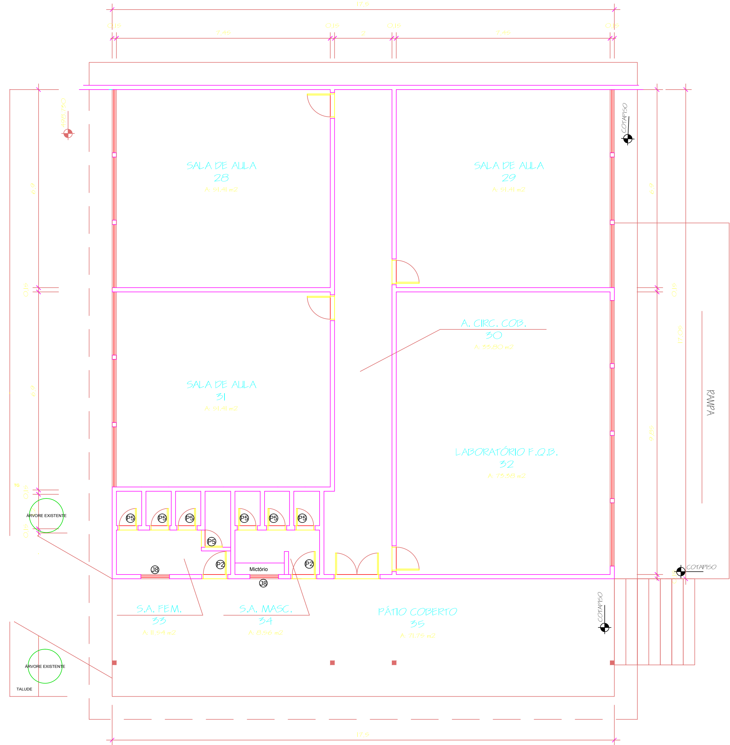
PLANTA BAIXA - BLOCO III Esc.: 1:75
