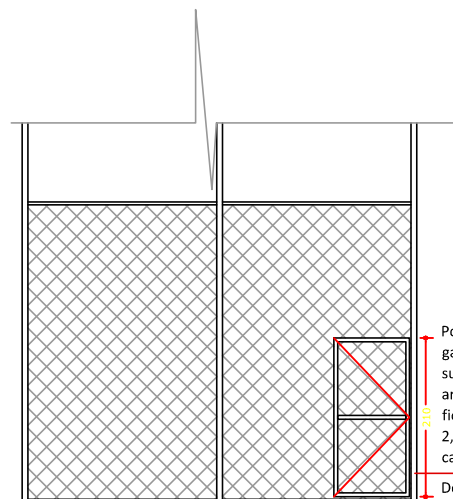
VISTA PORTÃO ACESSO
