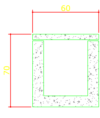
CORTE TRANSVERSAL CAIXA CAPTAÇÃO em Concreto sem escala
