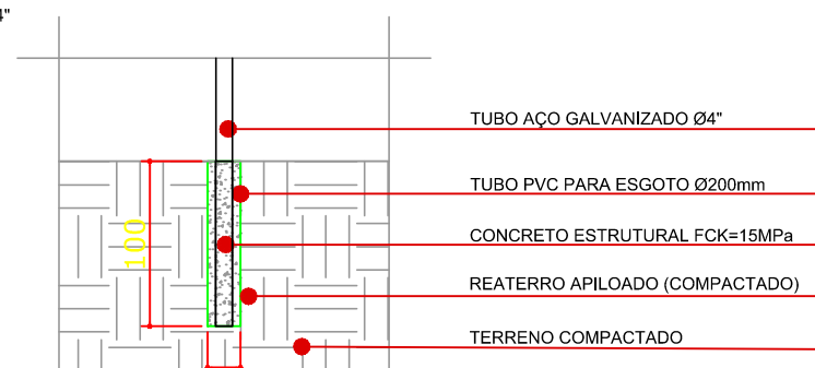
FUNDAÇÃO TRAVE sem escala
