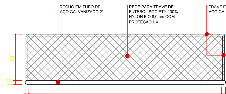
PLANTA TRAVE sem escala
