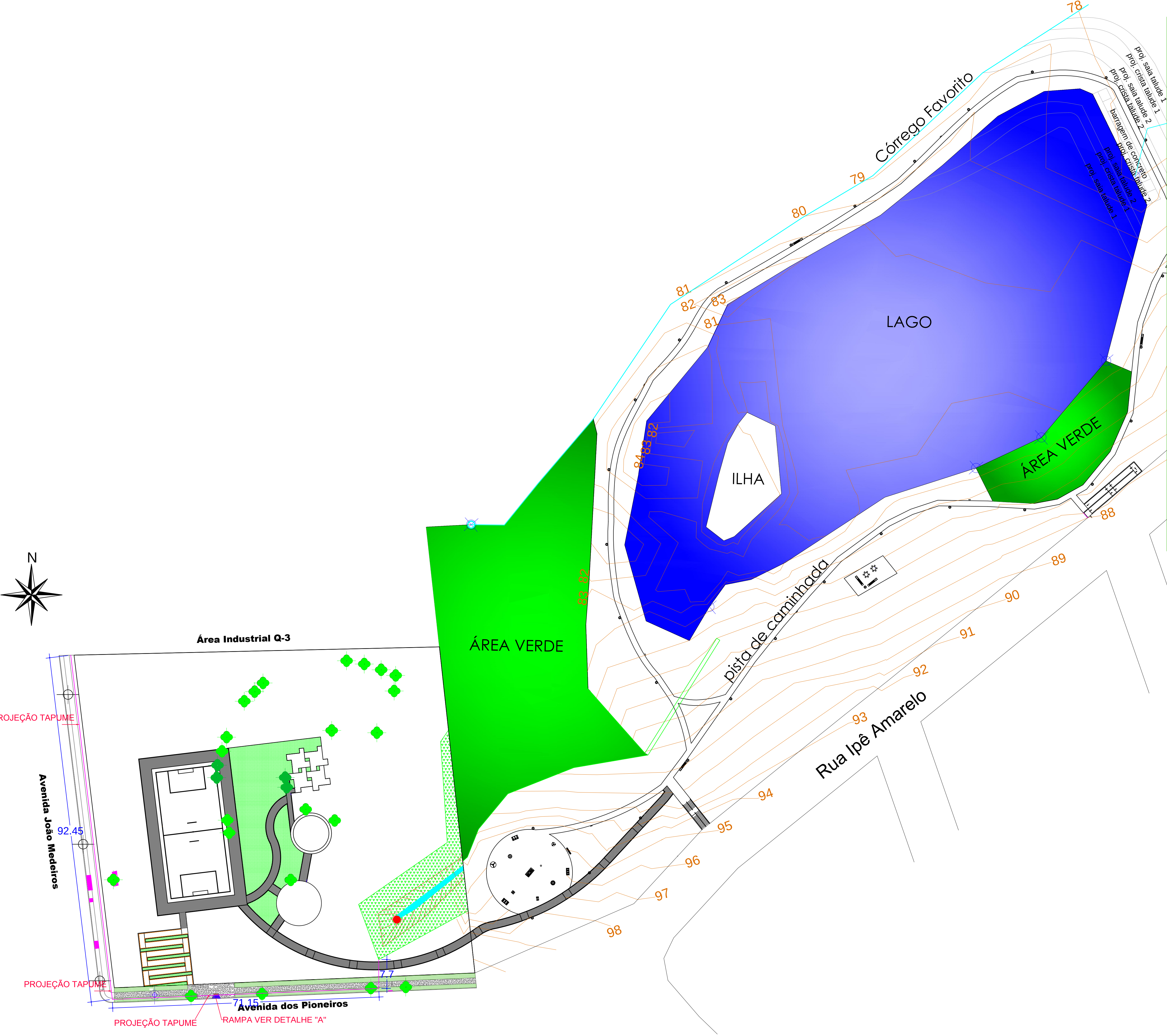
Planta de Implantação Geral Esc.: 1:500
