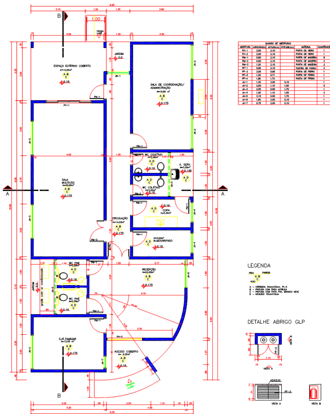
CRAS PORTE I E II - PLANTA BAIXA ÁREA: 165,30 m²
