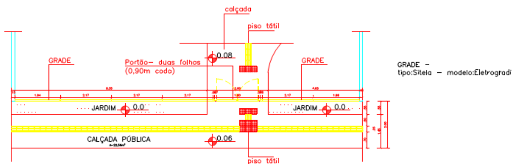
CRAS PORTE I E II - PLANTA BAIXA Grade, Portão e Calçada Pública - Área externa ÁREA: 185,30 m²
