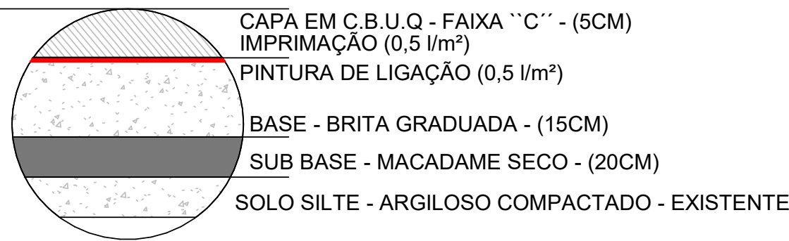
DETALHE PERFIL PAVIMENTAÇÃO EM C.B.U.Q. - RUA ROCHA POMBO 1 : 50
