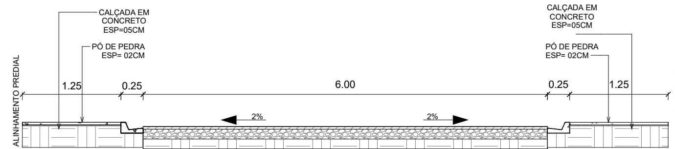
SEÇÃO TRANSVERSAL - TRECHO 01 AO 03 - ROCHA POMBO 1 : 75
