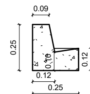
GUIA E SARJETA TIPO 02 DER 1 : 20
