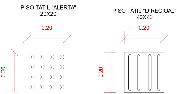
LEGENDA PISO TÁTIL 20X20 1 : 200
