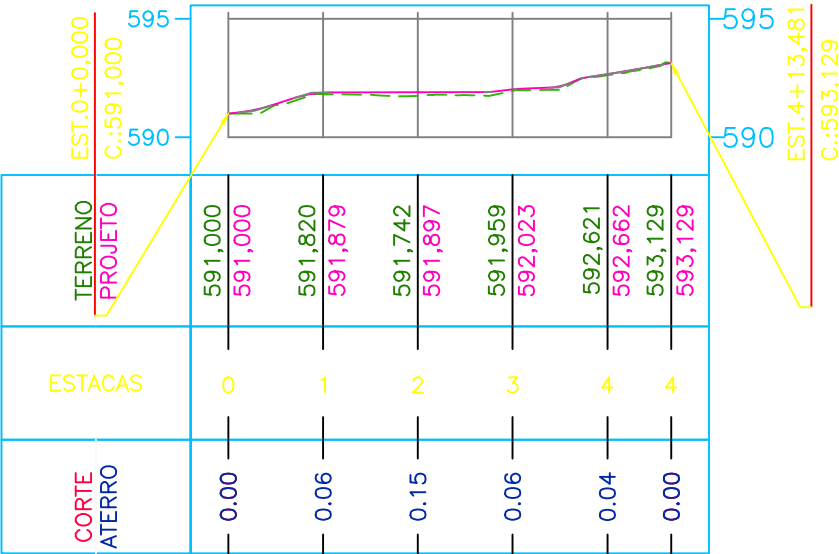
PERFIL LONGITUDINAL EIXO - RUA PAPOULA ESC. V.: 1:200
