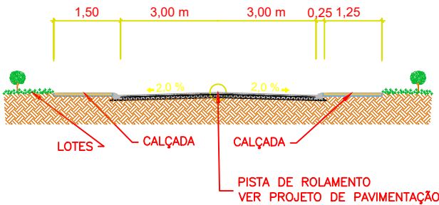
SEÇÃO TRANSVERSAL - TRECHO 01 - PAPOULA
