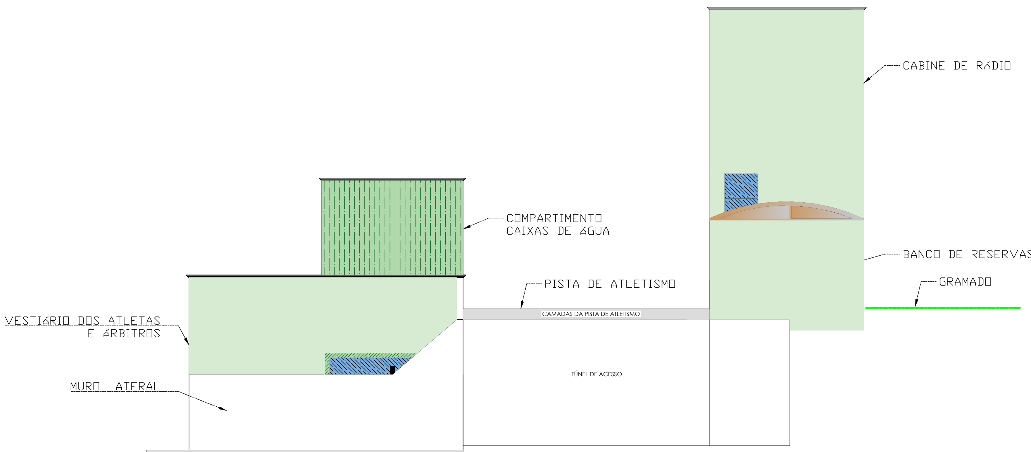
ELEVAÇÃO 02 ESCALA 1/50
