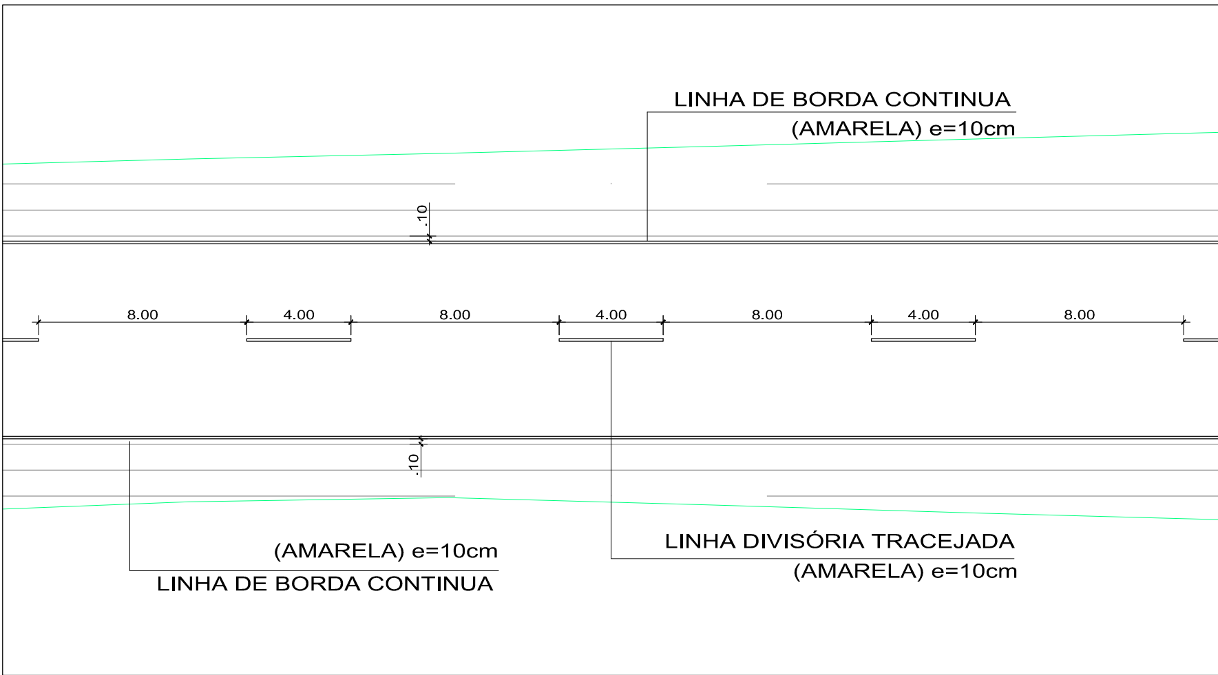
DETALHE SINALIZAÇÃO HORIZONTAL S/ ESCALA
