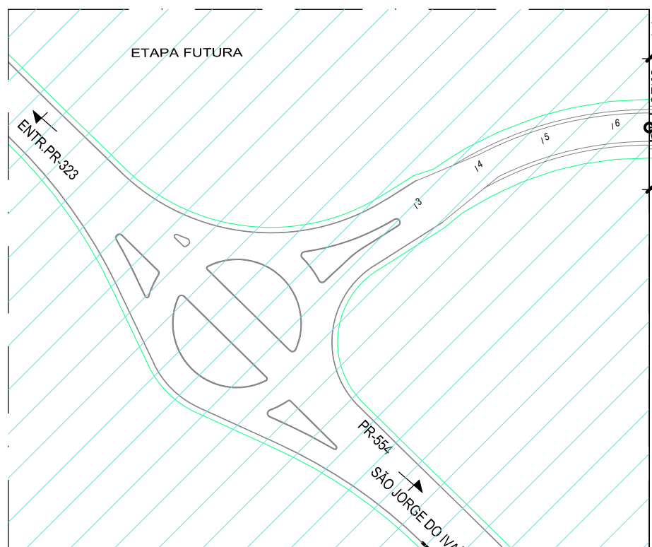
PROJETO SINALIZAÇÃO VIÁRIA ESCALA 1:1.500
