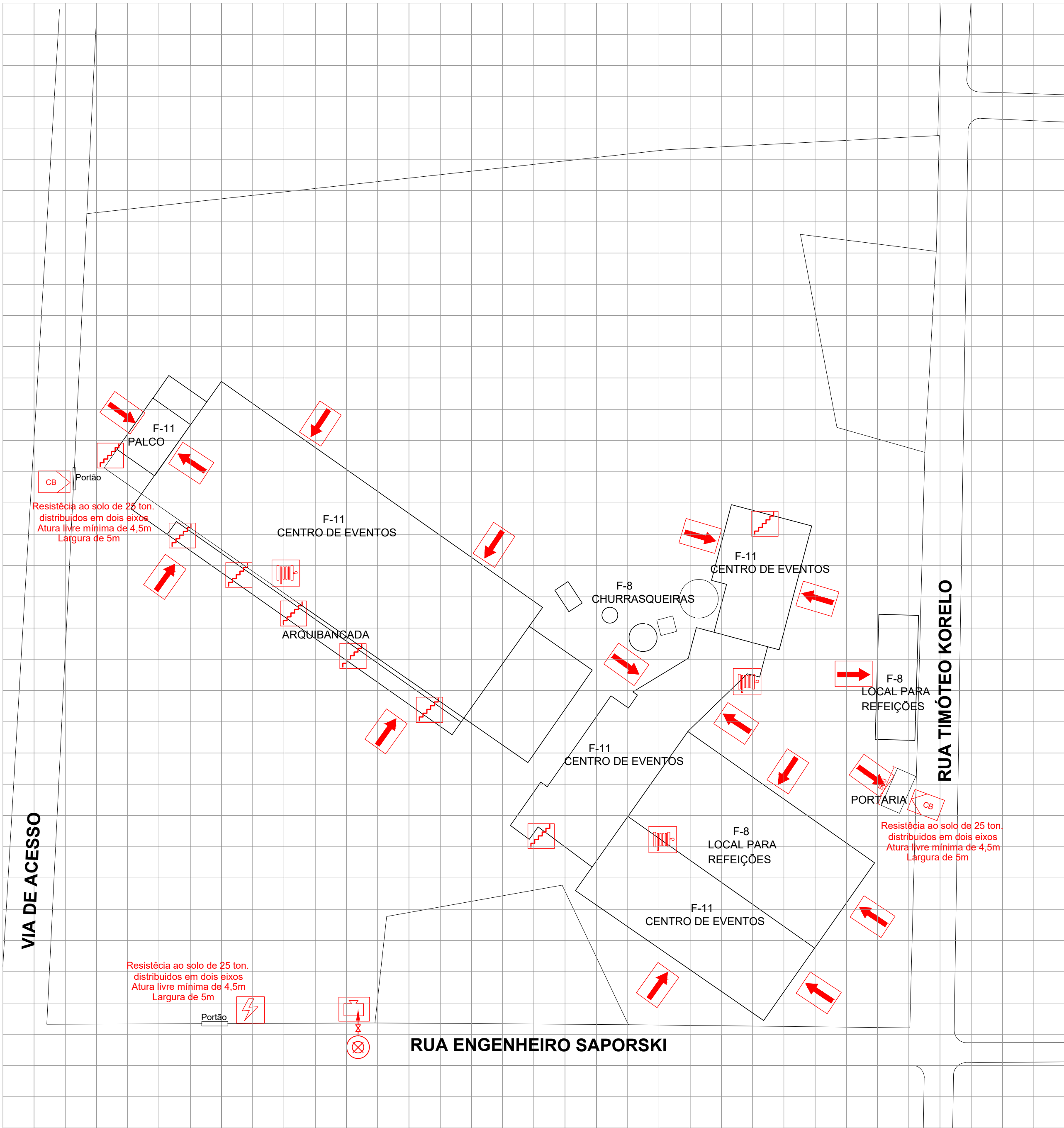
PLANTA DE RISCO DE INCÊNDIO
