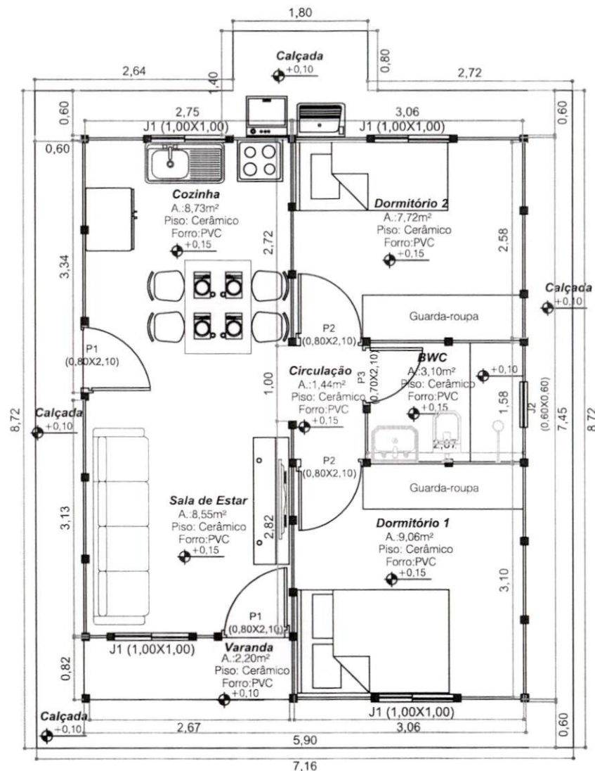
PLANTA BAIXA ESCALA: 1/50
