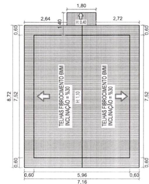
PLANTA DE COBERTURA ESCALA: 1/100
