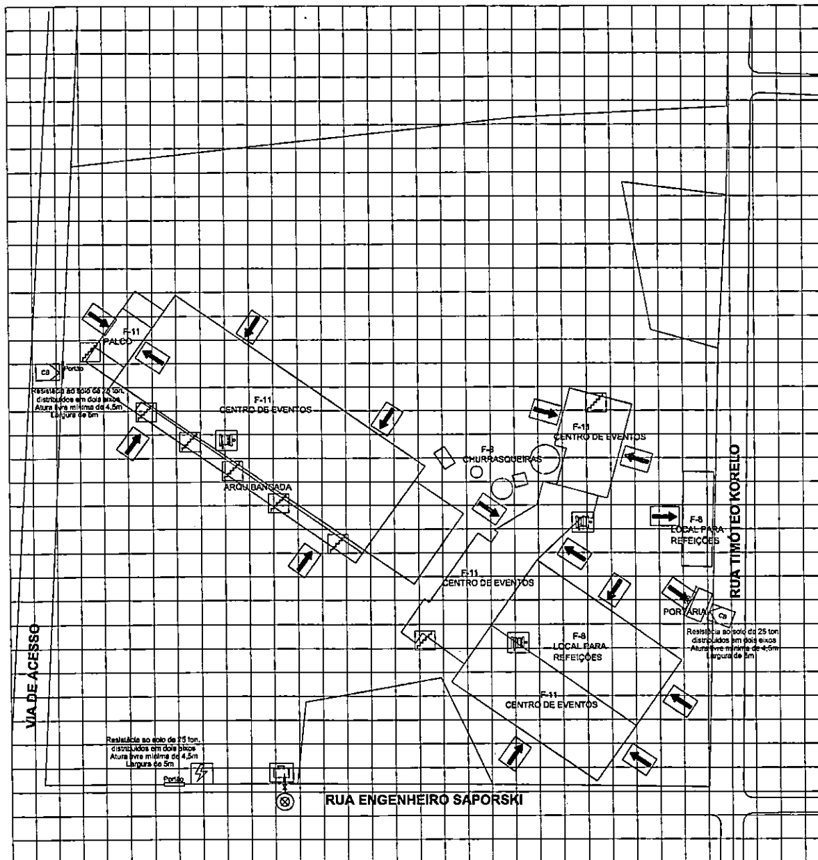
PLANTA DE RISCO DE INCÊNDIO Escala 1:1.000
