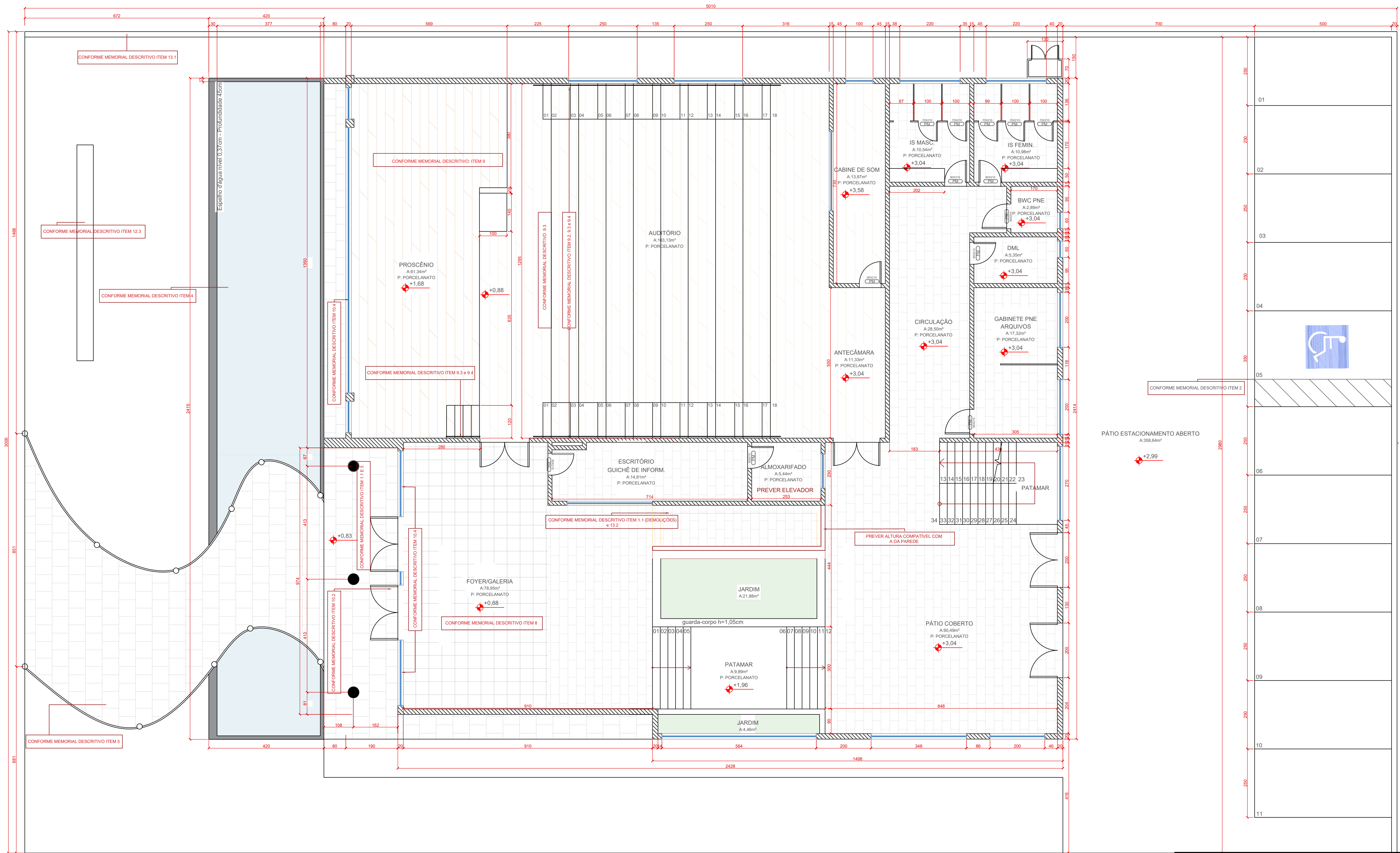
PLANTA PAVIMENTO TÉRREO ÁREA TOTAL = 630,21m² ESC 1/75
