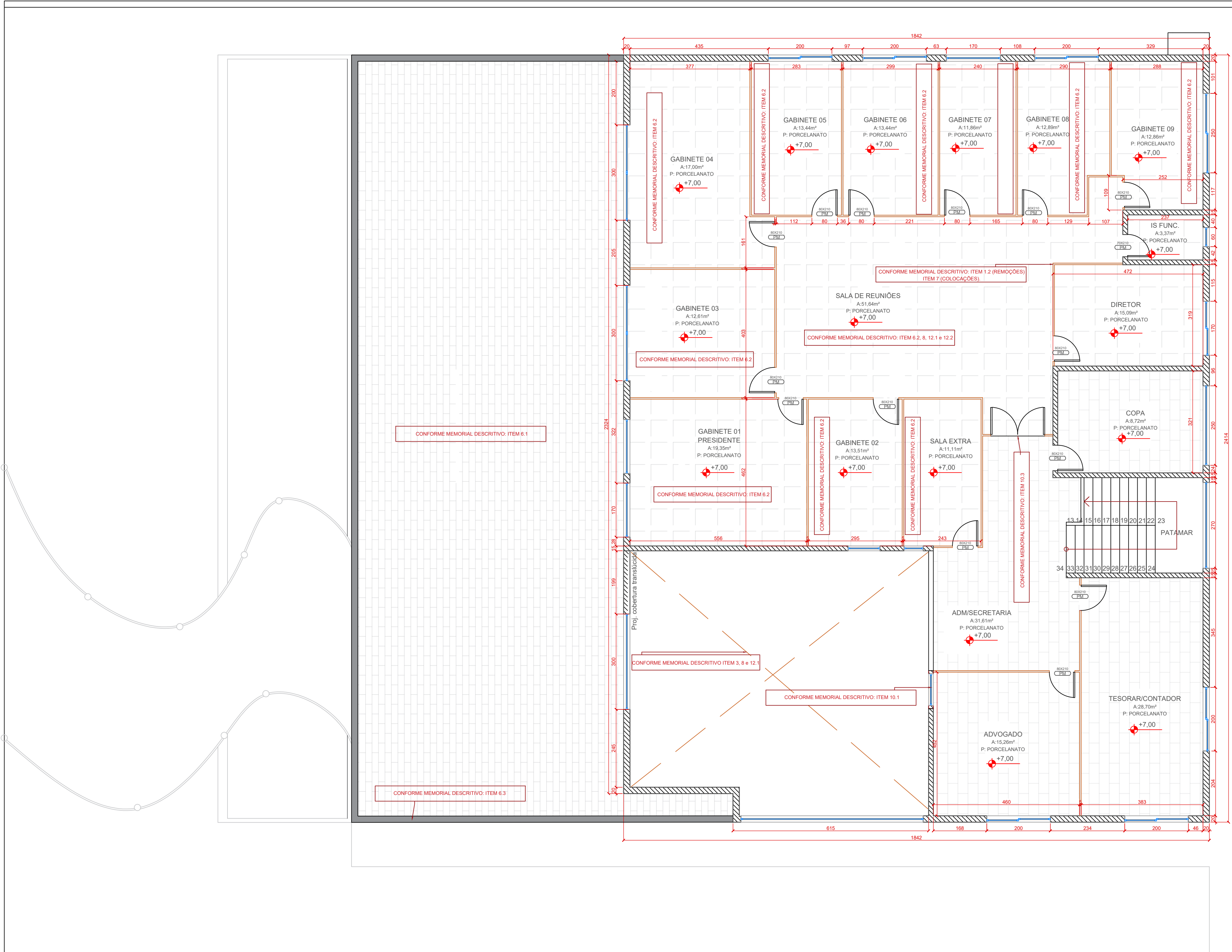
PLANTA PAVIMENTO SUPERIOR ÁREA TOTAL = 352,79m² ESC: 1:75
