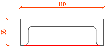
DETALHE DA BOCA-DE-LOBO VISTA FRONTAL
