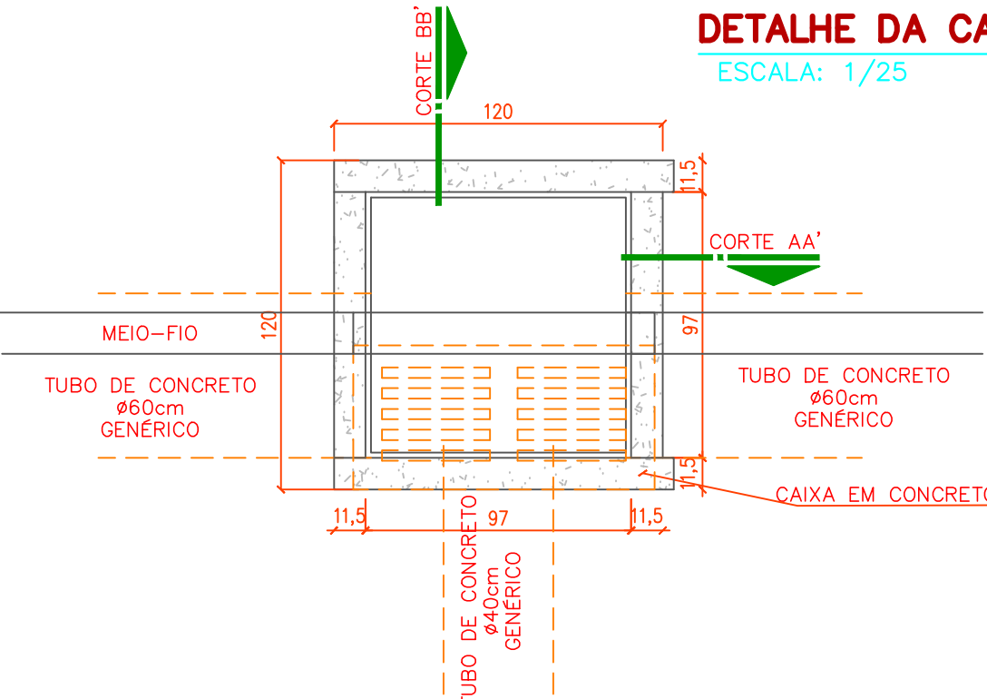
DETALHE DO CORPO DA CAIXA PLANTA
