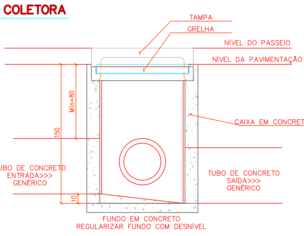
CORTE A
