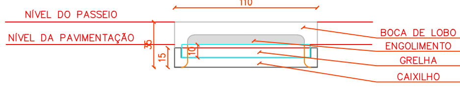
MONTAGEM VISTA FRONTAL
