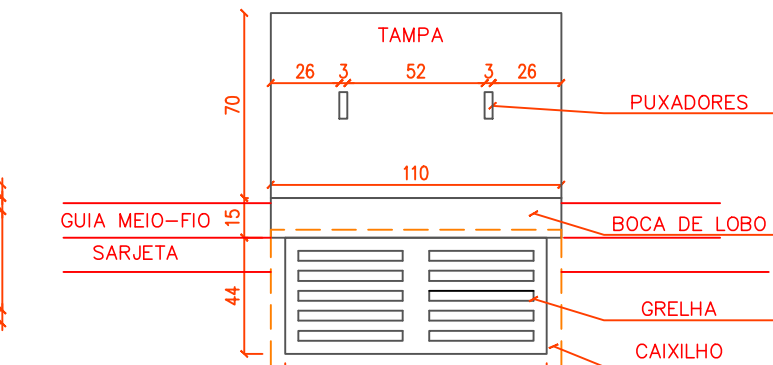
DETALHE DA GRELHA PLANTA
