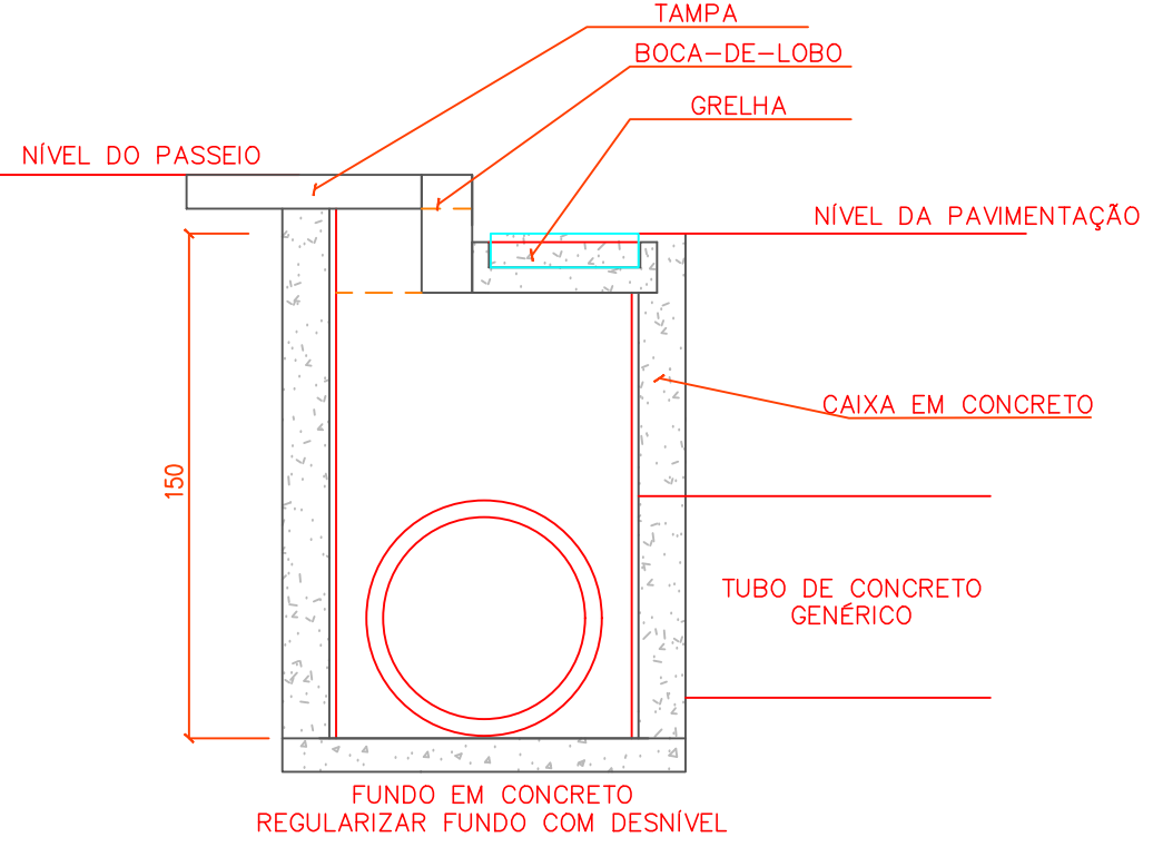
CORTE B
